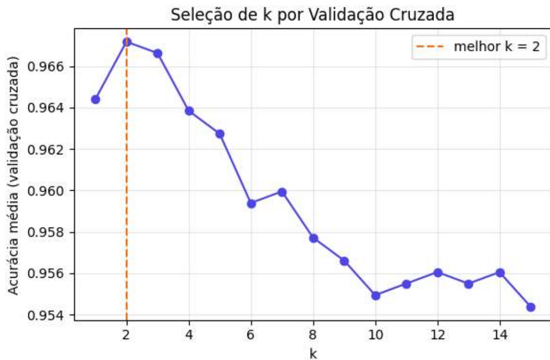
Figura 7.16: Acurácia média por validação cruzada (5 partições) em função do parâmetro k , para a base de dígitos com vetores de intensidade brutos.
