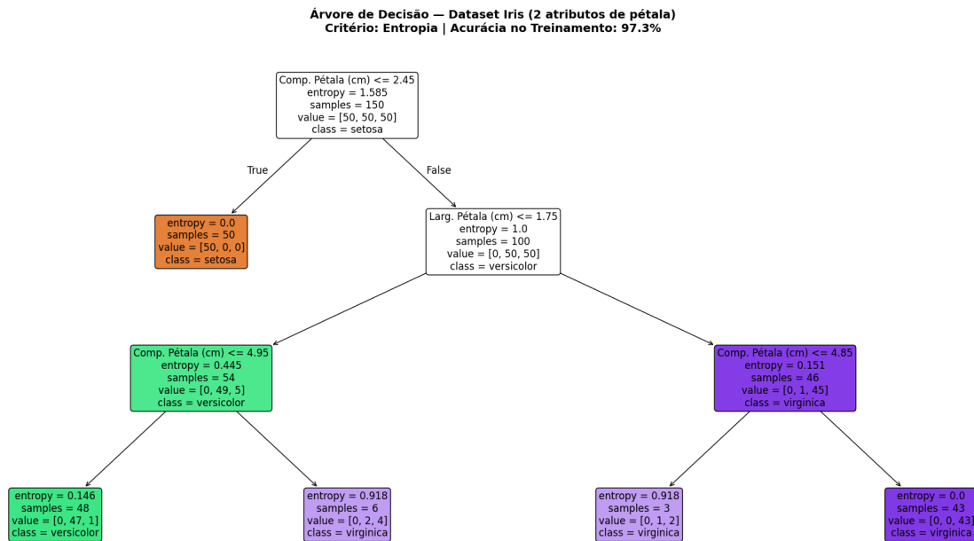
Figura 3.25: Árvore de Decisão treinada com Scikit-learn no dataset Iris (apenas pétalas).
