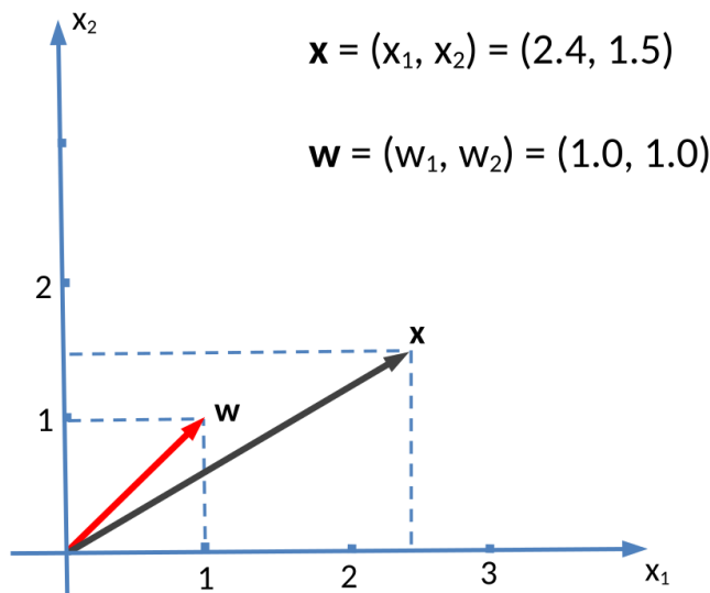
Figura 5.11: Produto Interno dos Vetores \mathbf{w} e \mathbf{x} .
