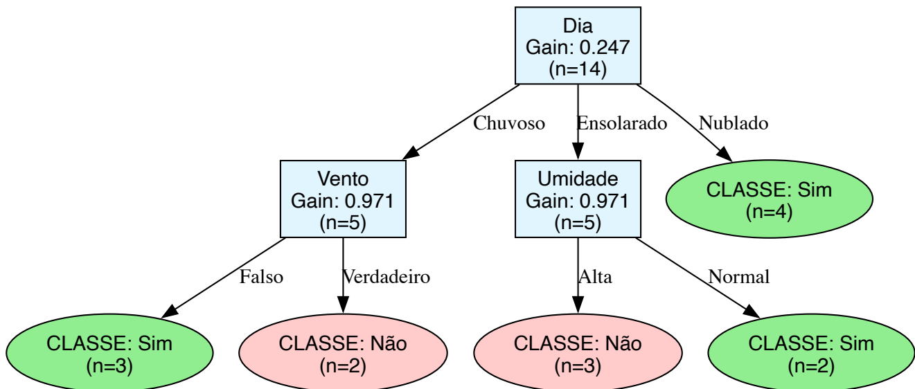
Figura 3.22: Árvore de Decisão ID3 construída sobre a Tabela do Tempo.
