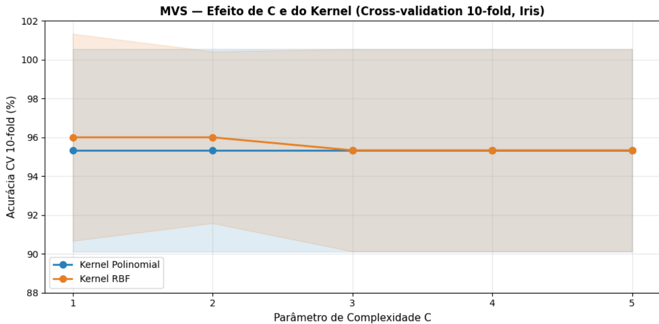
Figura 5.27: Cross-validation 10-fold com MVS — Efeito de C e do Kernel no Dataset Iris.
