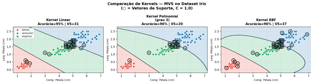
Figura 5.26: Comparação de Kernels da MVS no Dataset Iris (atributos de pétala).
