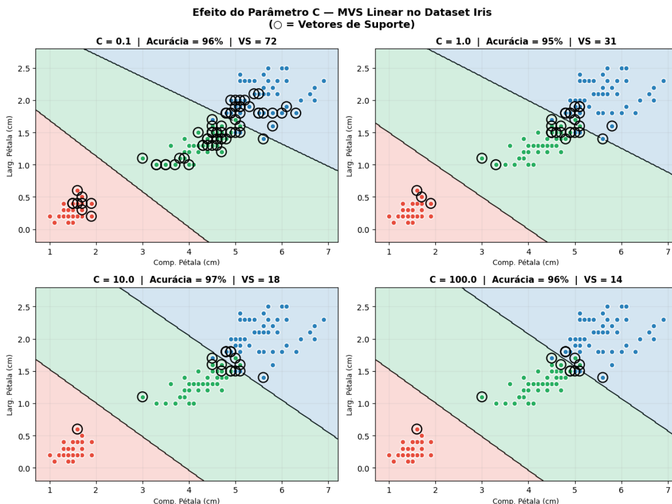
Figura 5.25: Efeito do Parâmetro C nas Bordas de Decisão da MVS (Iris, kernel linear).
