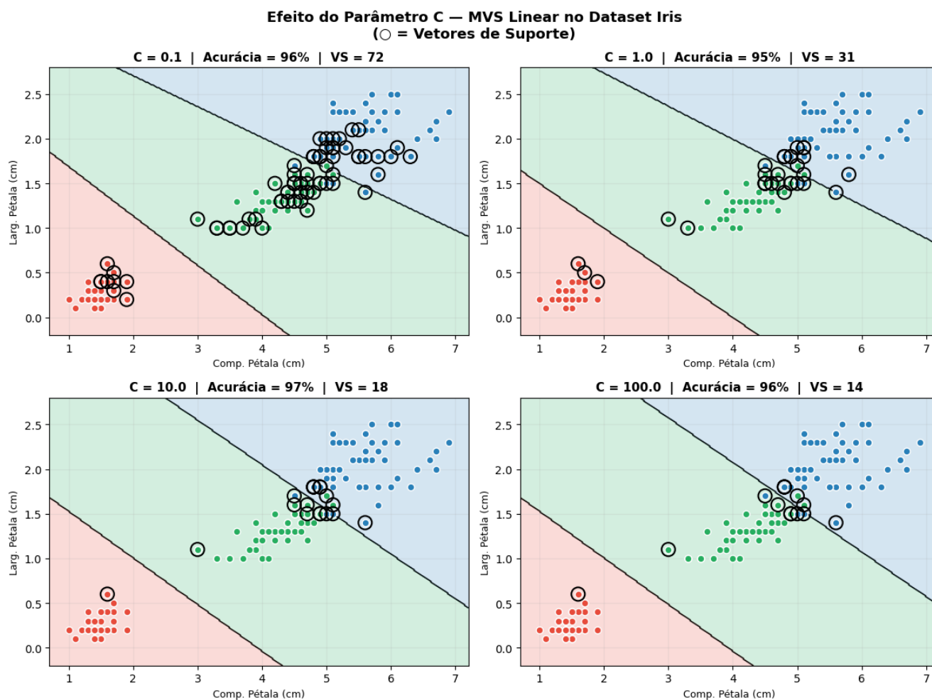
Figura 5.24: Efeito do Parâmetro C nas Bordas de Decisão da MVS (Iris, kernel linear).
