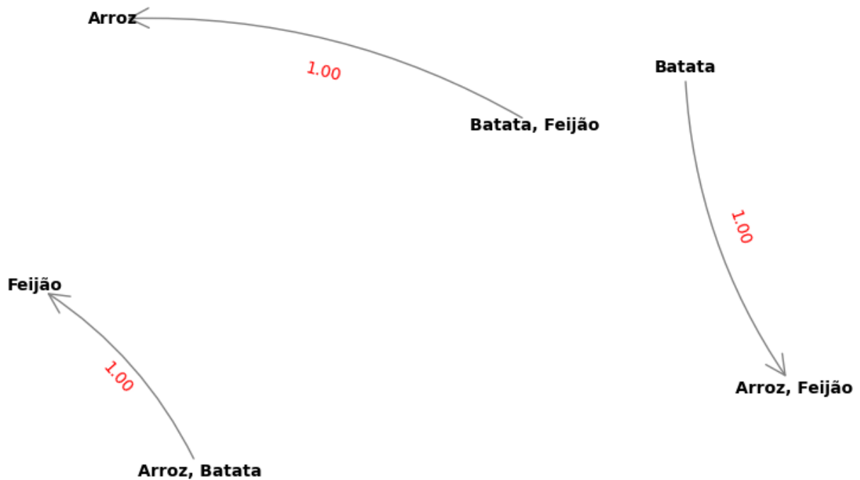
Figura 2.14: Grafo de associação: setas indicam a direção da regra e valores representam a confiança ( \text{conf\_min}=0.9 ).
