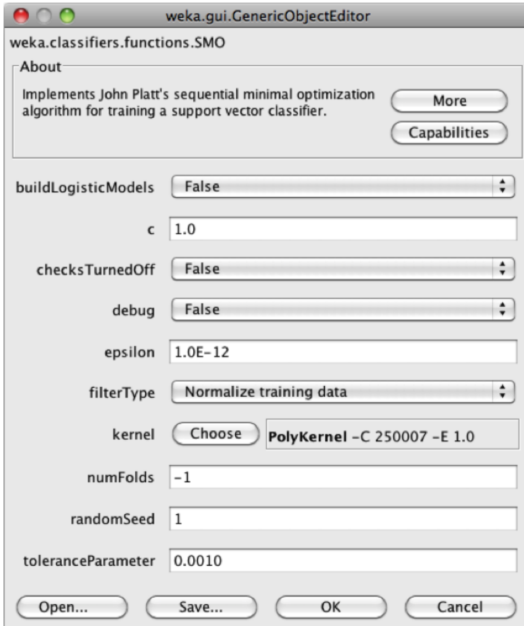
Figura 5.19: Janela de Ajustes de Parâmetros do SMO.
