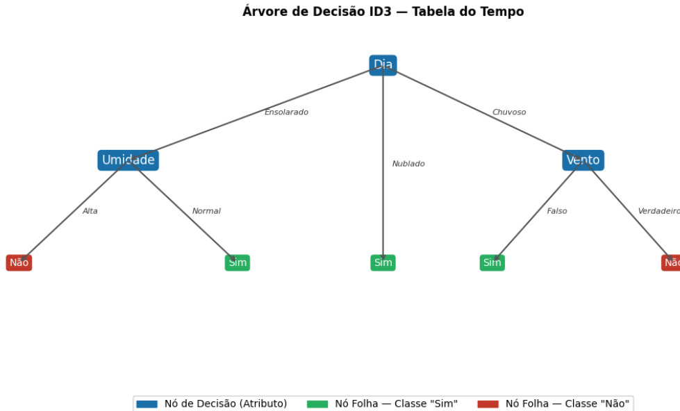
Figura 3.22: Árvore de Decisão ID3 construída sobre a Tabela do Tempo.
