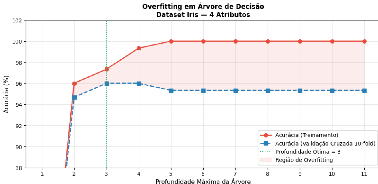
Figura 3.26: Overfitting: Acurácia de Treinamento vs. Validação Cruzada por Profundidade.
