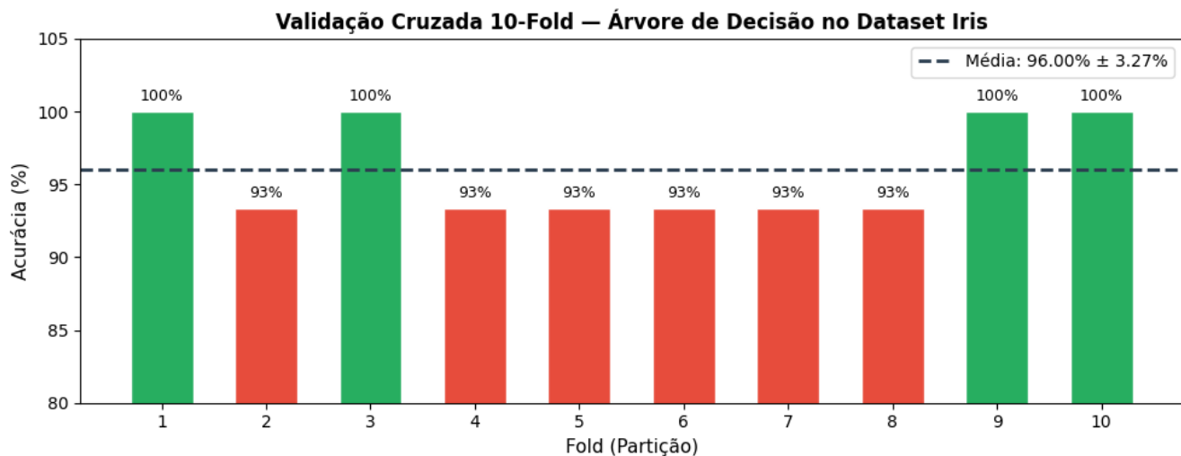
Figura 3.25: Validação Cruzada (10-fold) — Acurácia por Partição.
