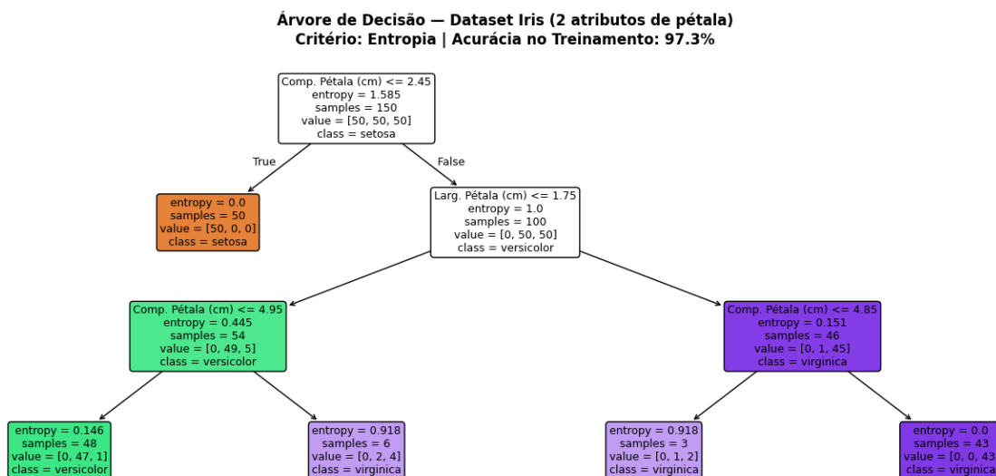
Figura 3.24: Árvore de Decisão treinada com Scikit-learn no dataset Iris (apenas pétalas).
