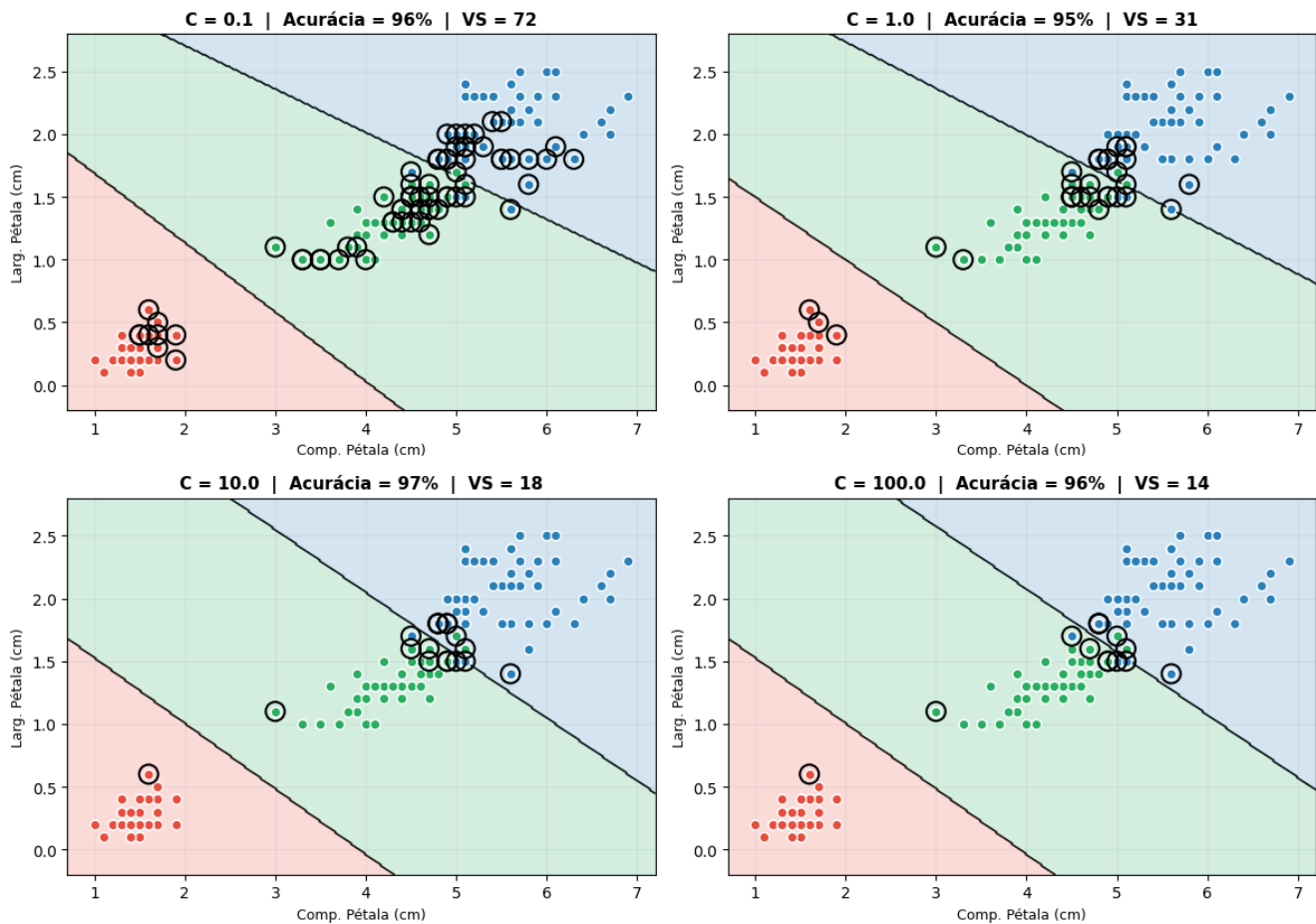
Figura 5.24: Efeito do Parâmetro C nas Bordas de Decisão da MVS (Iris, kernel linear).
