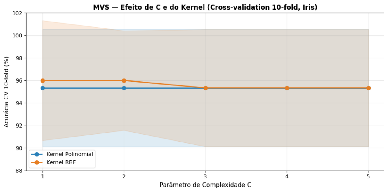
Figura 5.26: Cross-validation 10-fold com MVS — Efeito de C e do Kernel no Dataset Iris.
