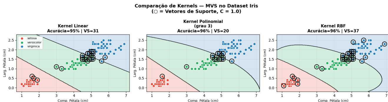
Figura 5.25: Comparação de Kernels da MVS no Dataset Iris (atributos de pétala).
