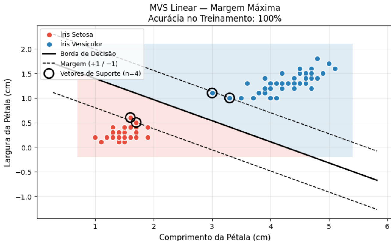
Figura 5.23: MVS Linear — Margem Máxima entre Íris Setosa e Versicolor (atributos de pétala).
