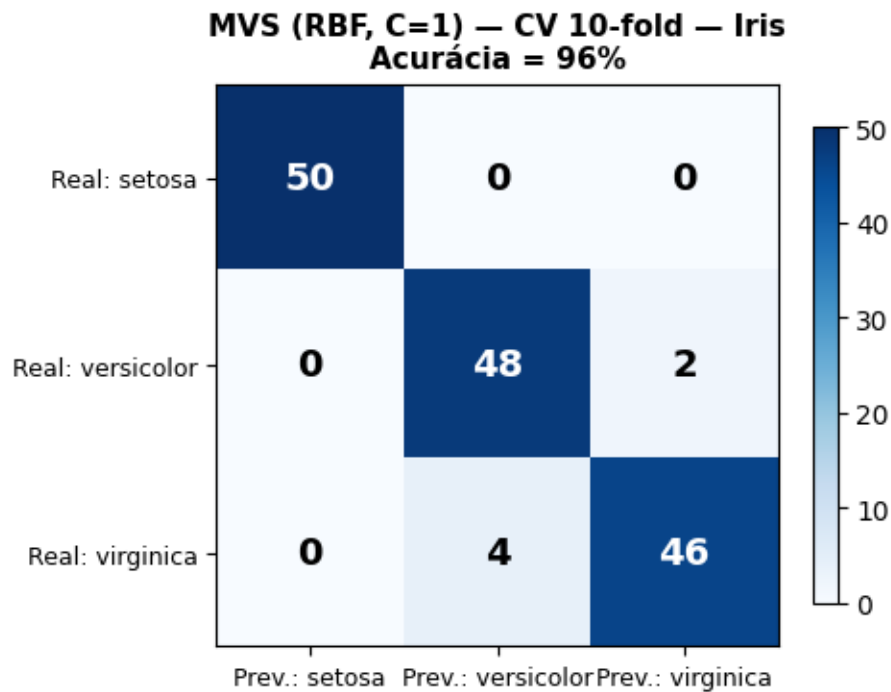
Figura 5.27: Matriz de Confusão — MVS RBF C=1 com Cross-validation 10-fold no Iris.
