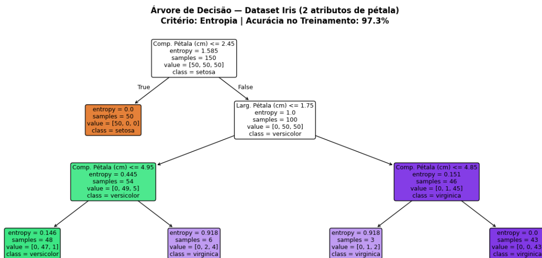
Figura 3.25: Árvore de Decisão treinada com Scikit-learn no dataset Iris (apenas pétalas).
