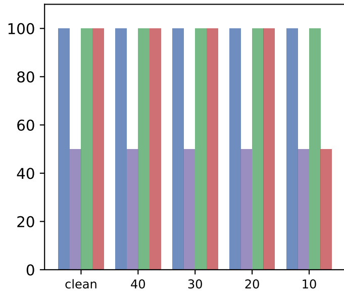
KdV
