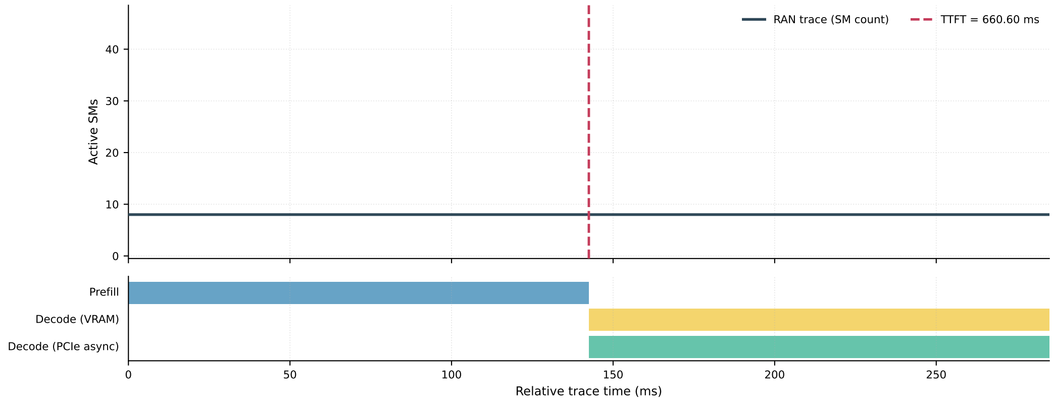
RAN trace interleaving exemplar · OPT-2.7B · N=256 · L=8192
