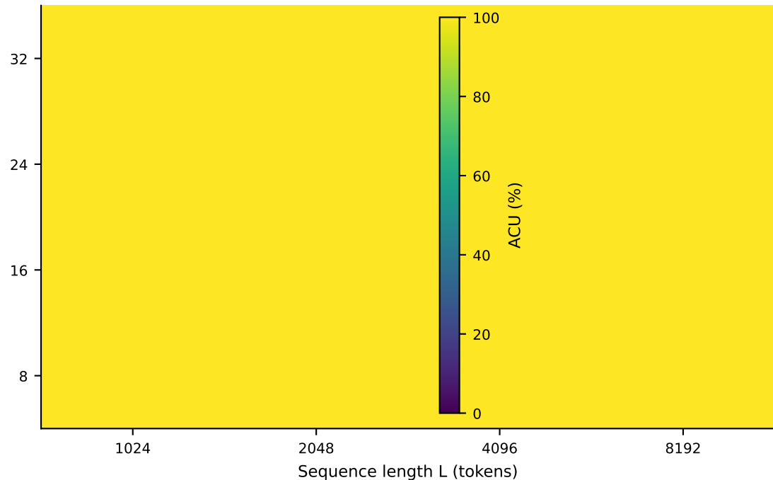
OPT-2.7B · Decode
