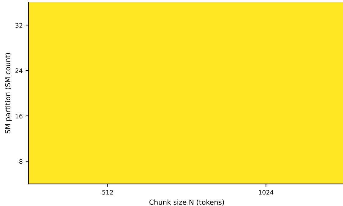
OPT-2.7B · Prefill
