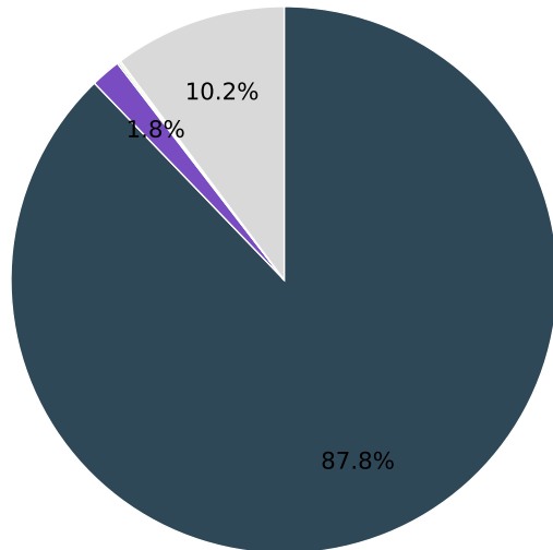
OPT-6.7B · N=512
