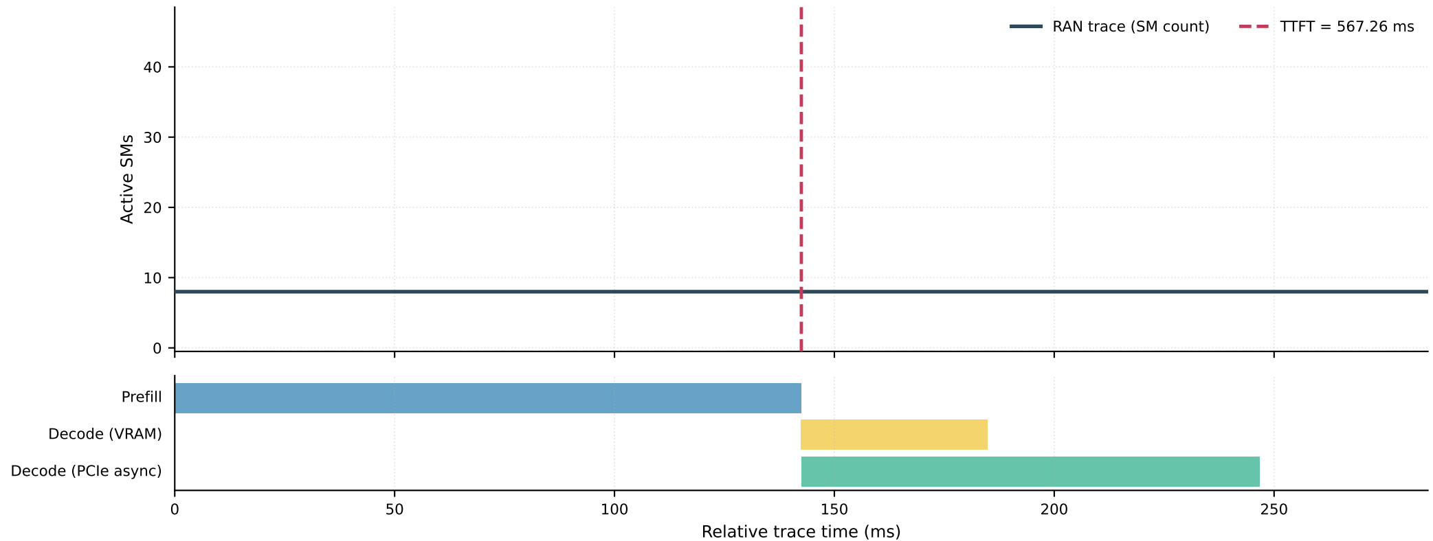
RAN trace interleaving exemplar · OPT-125M · N=64 · L=1024
