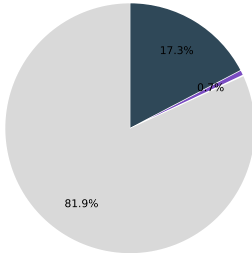
OPT-1.3B · N=512
