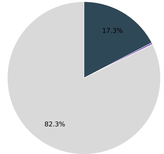
OPT-1.3B · N=256
