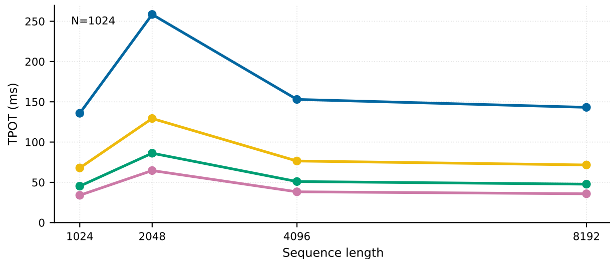
OPT-2.7B · DGX VRAM fetch
