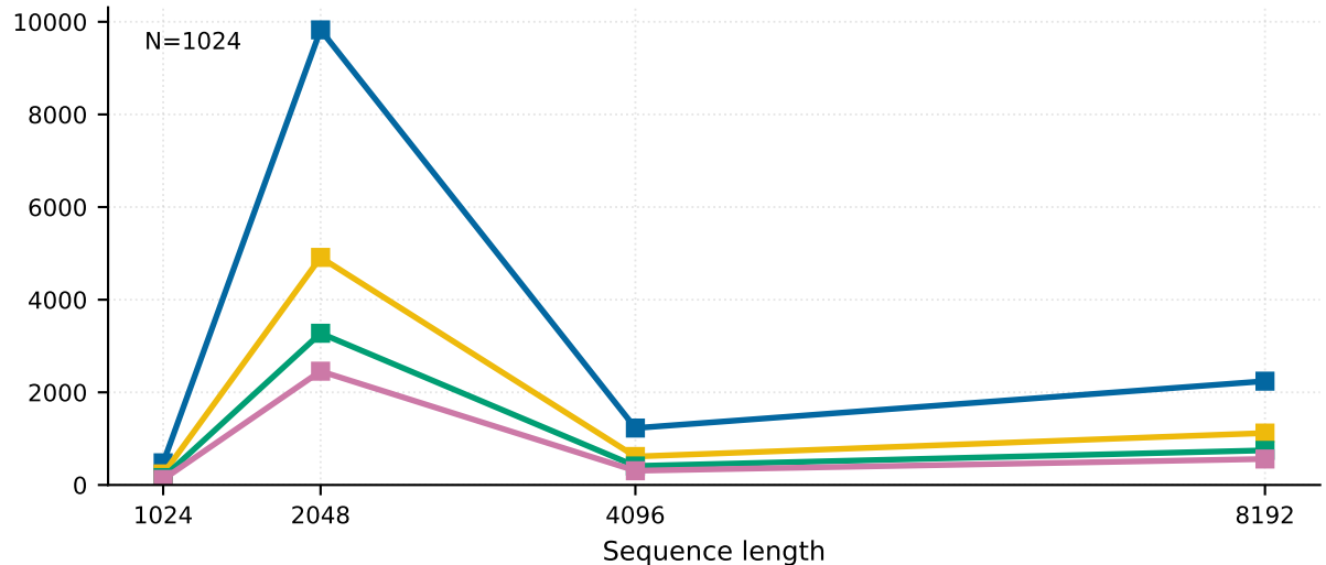
OPT-6.7B · PCIe async fetch
