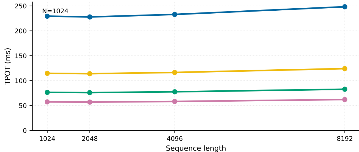
OPT-6.7B · DGX VRAM fetch
