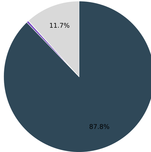
OPT-6.7B · N=1024
