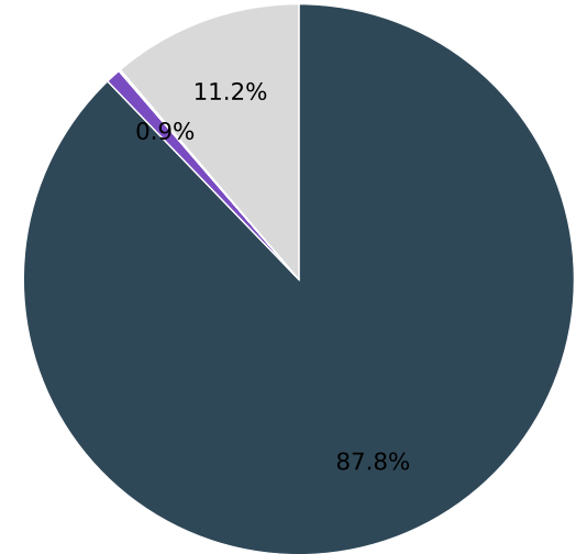
OPT-6.7B · N=256
