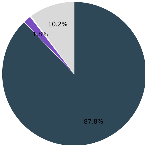
OPT-6.7B · N=512
