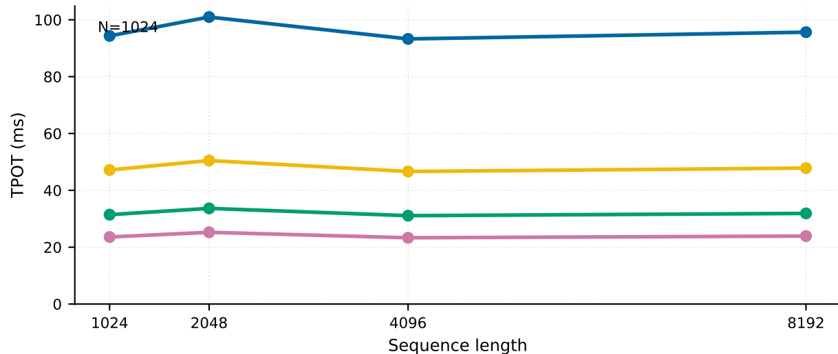
OPT-350M · DGX VRAM fetch
