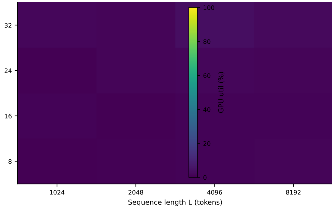
OPT-350M · Decode
