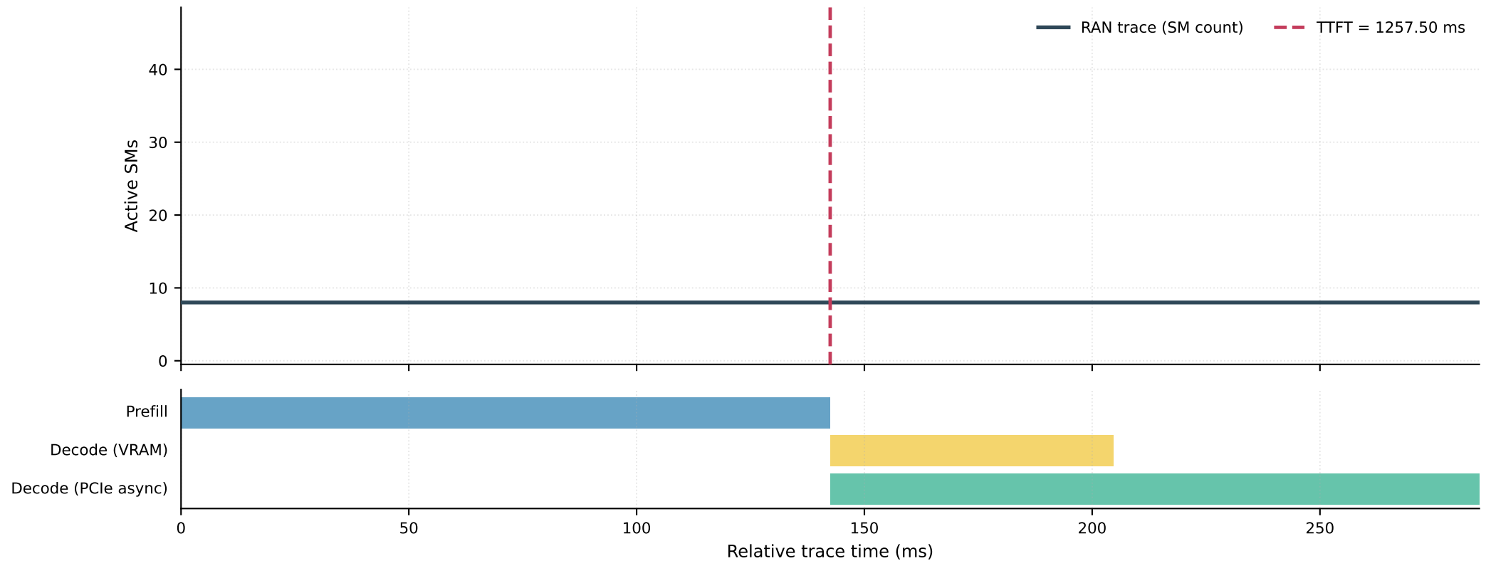
RAN trace interleaving exemplar · OPT-6.7B · N=1024 · L=8192
