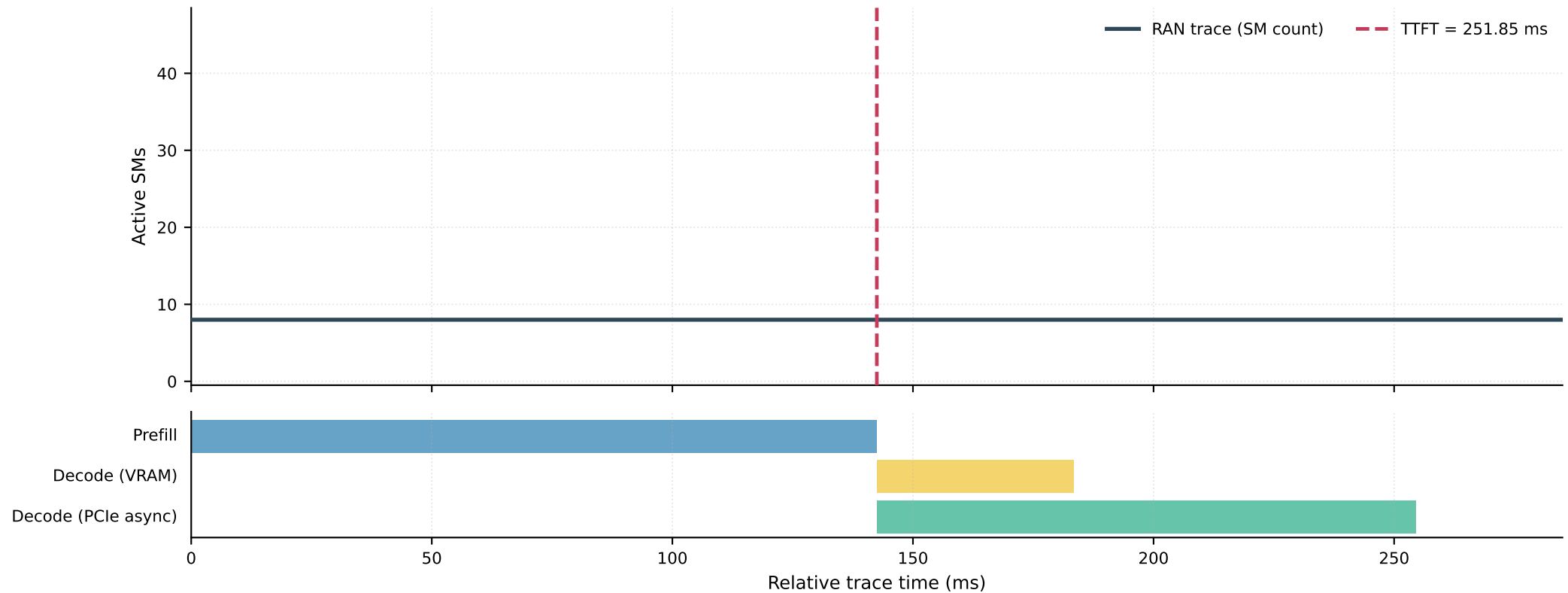
RAN trace interleaving exemplar · OPT-1.3B · N=1024 · L=8192
