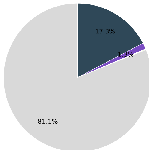
OPT-1.3B · N=1024
