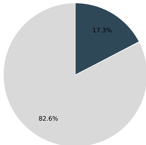
OPT-1.3B · N=512
