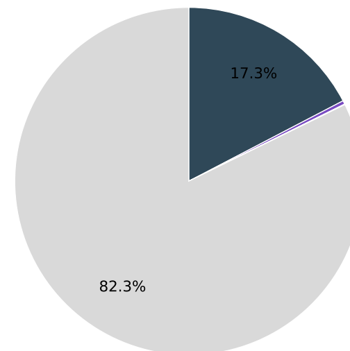
OPT-1.3B · N=256
