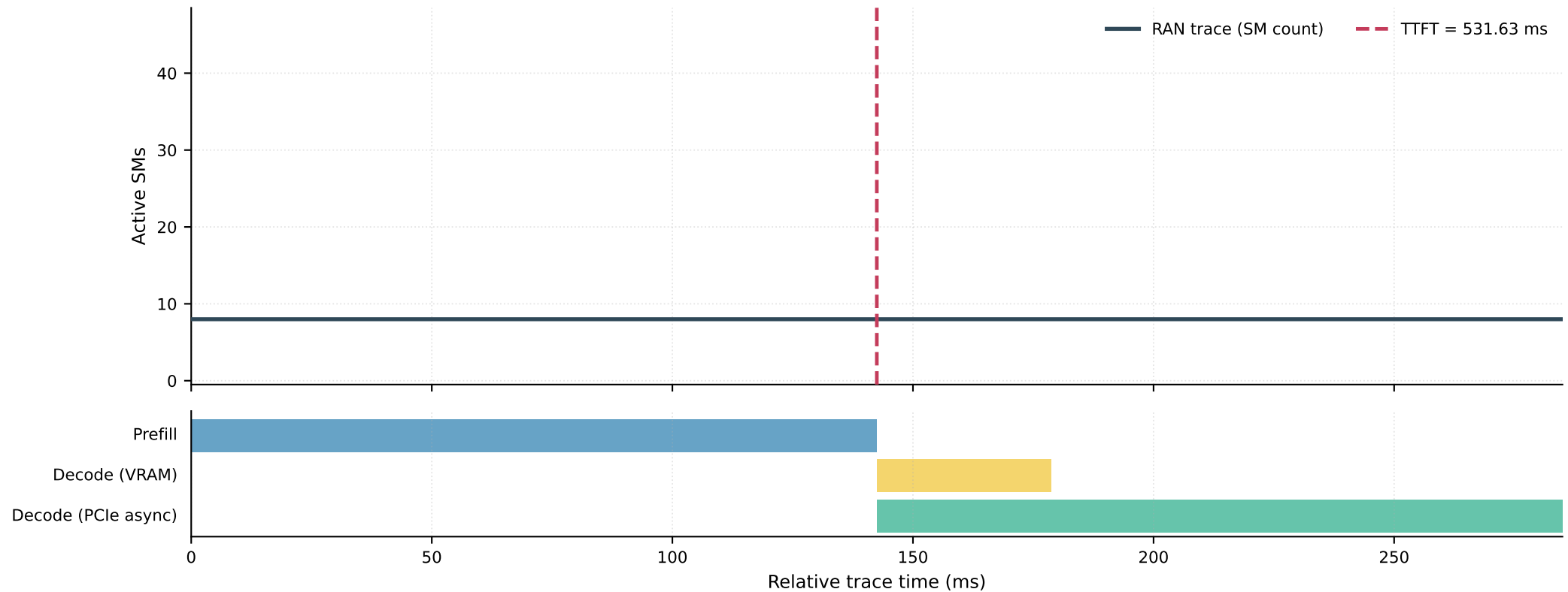
RAN trace interleaving exemplar · OPT-2.7B · N=1024 · L=8192
