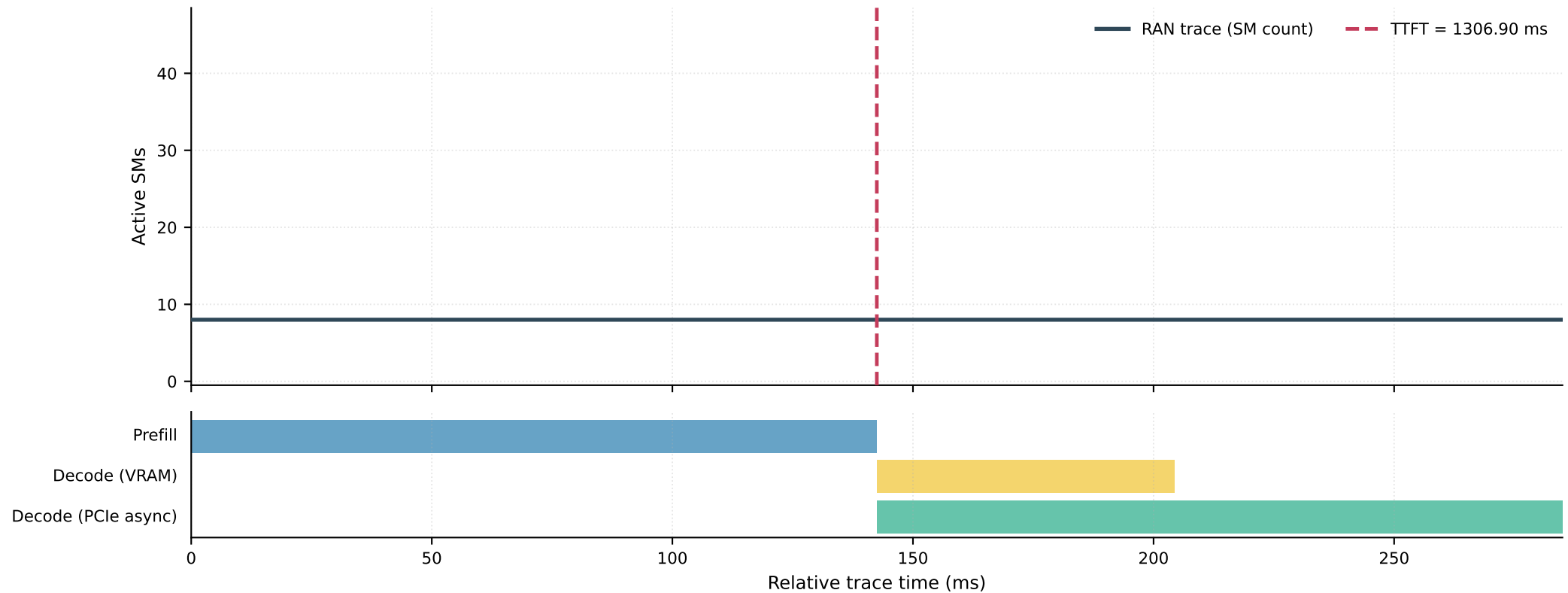
RAN trace interleaving exemplar · OPT-6.7B · N=512 · L=8192
