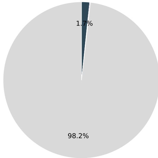
OPT-125M · N=512
