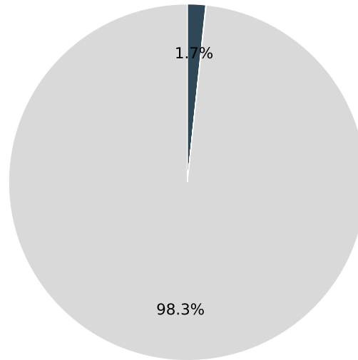
OPT-125M · N=1024
