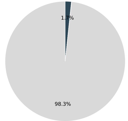
OPT-125M · N=256
