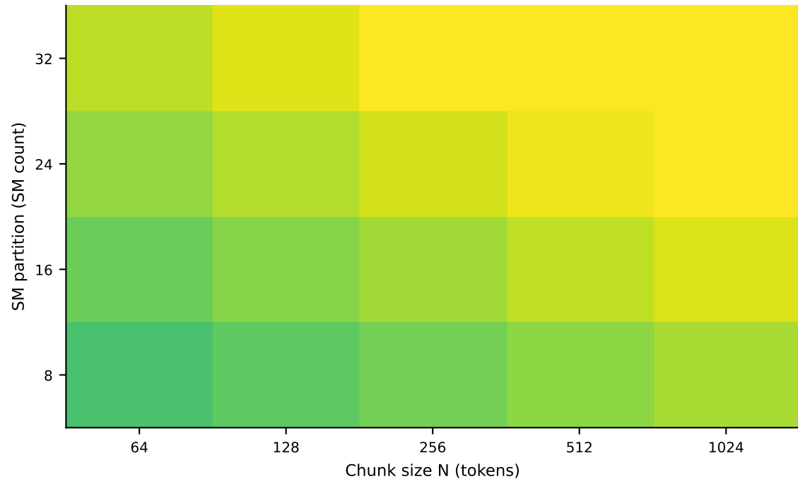
OPT-125M · Prefill
