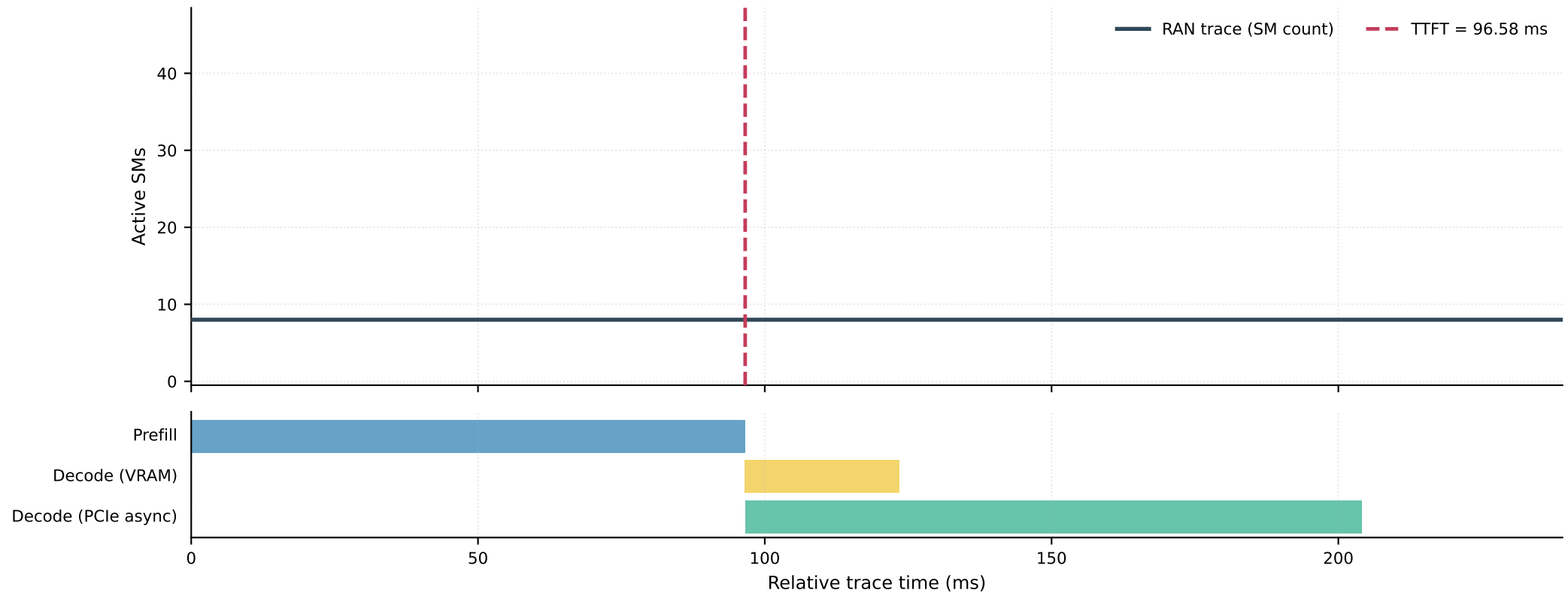
RAN trace interleaving exemplar · OPT-350M · N=1024 · L=8192
