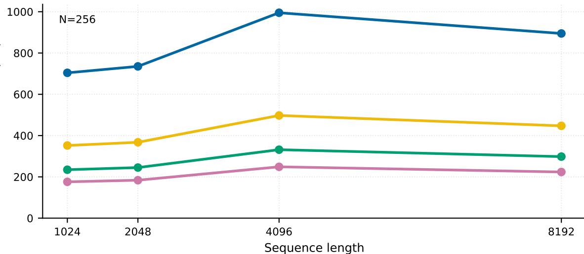
OPT-1.3B · DGX VRAM fetch
