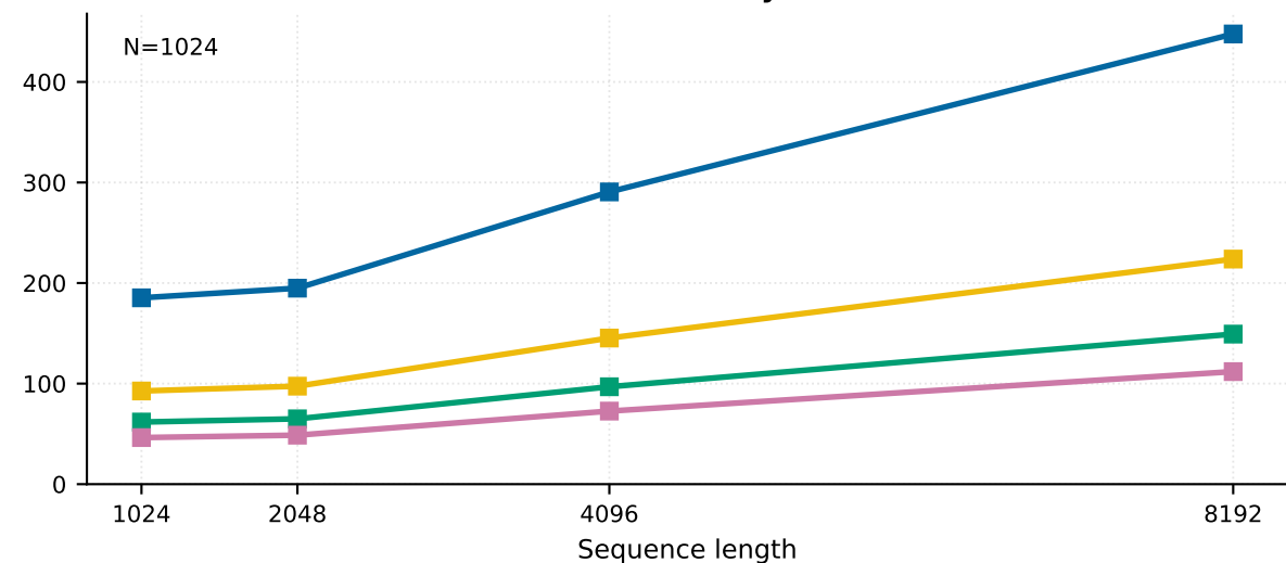
OPT-1.3B · PCIe async fetch
