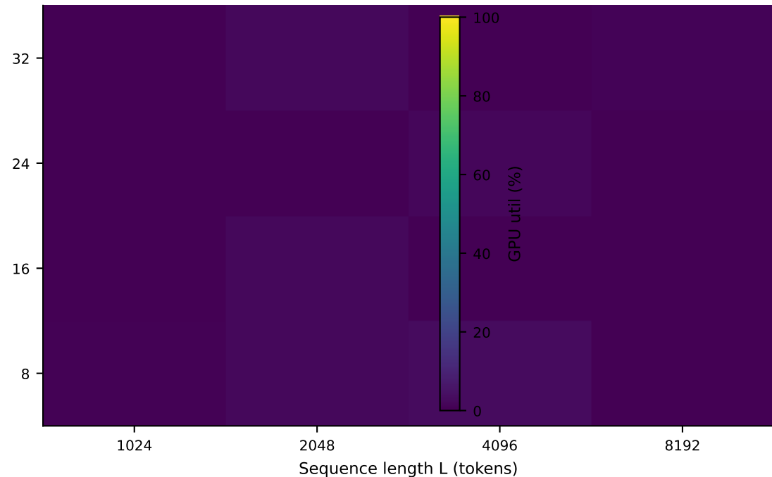
OPT-1.3B · Decode
