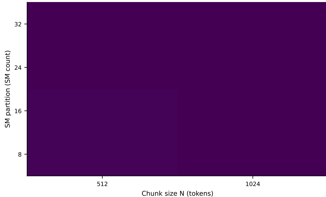
OPT-1.3B · Prefill
