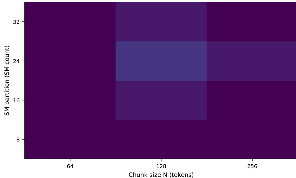
OPT-6.7B · Prefill
