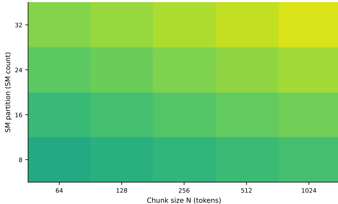
OPT-350M · Prefill
