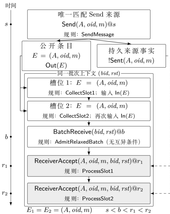
图2 无互异约束模型中的重复接受可达执行
