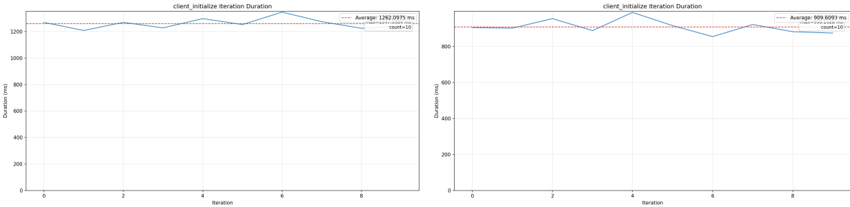
图 2: client_initialize 基准的单次迭代耗时对比。左图为优化前，右图为优化后。可以看到优化后整条曲线整体下移，平均值和峰值均明显降低。
