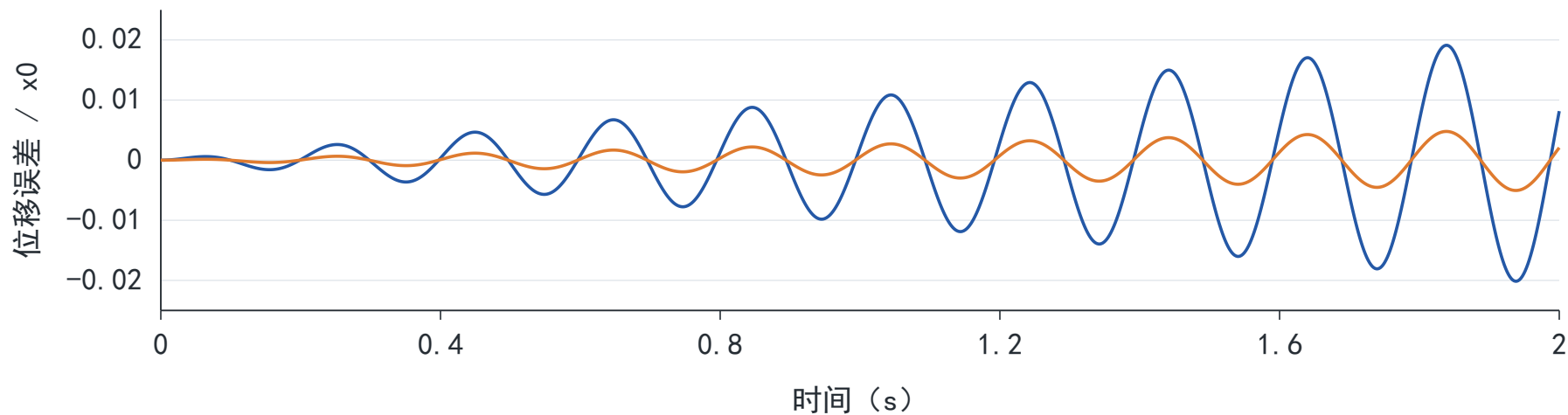
(b) 零物理阻尼下的位移相位误差
