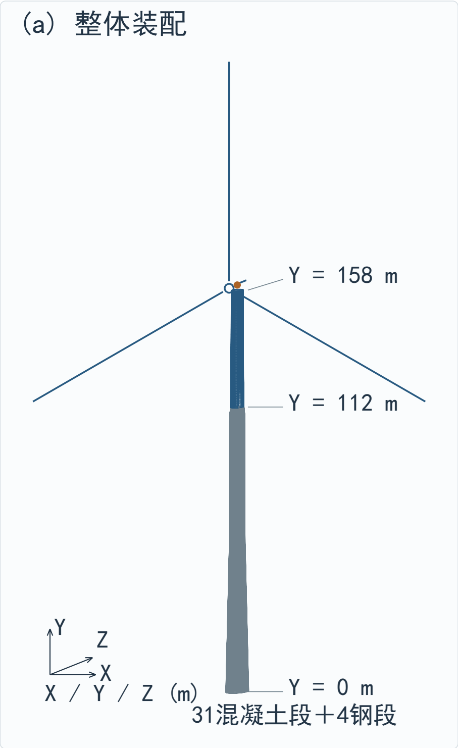
图2-1 塔架与刚体RNA输入几何 依据M2实际节点与单元连接绘制；未变形几何，坐标单位m。
