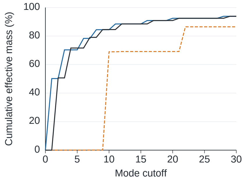
(d) M3 modal mass participation
