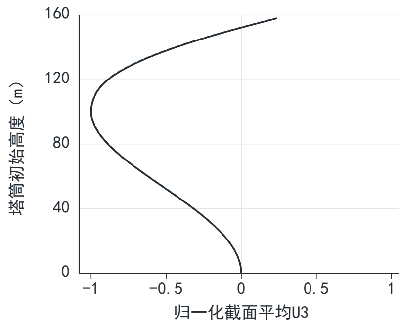
(d) 第4阶 (Z) : 0.74244 Hz
