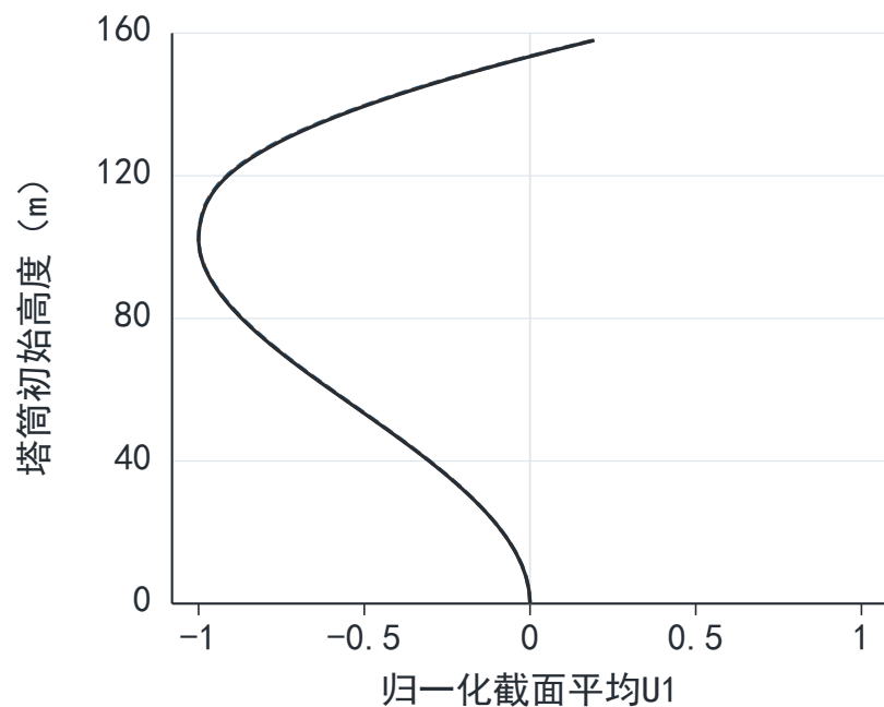
(c) 第3阶 (X) : 0.70763 Hz
