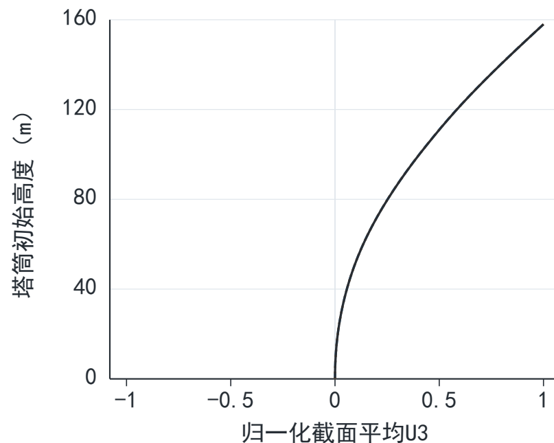
(d) 第4阶 (Z) : 0.74244 Hz
