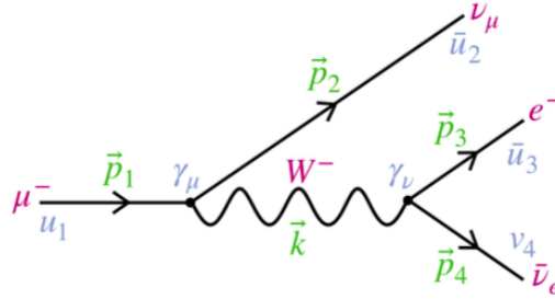
Figure 5.2: Processo di decadimento del muone.
