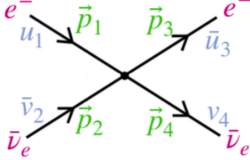
Figure 5.1: Rappresentazione processo e + \bar{\nu}_e \longrightarrow e + \bar{\nu}_e .
