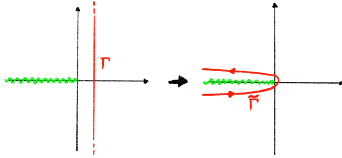
Figura 4.14: Cammini di integrazione \Gamma e \tilde{\Gamma} .
