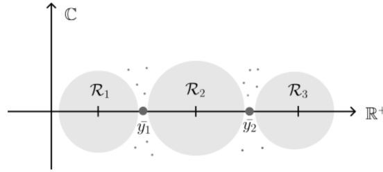
Figura 6.2: Nota che il fatto che la regione R_3 sia una circonferenza e nella figura 6.3 una curva aperta è solo un problema di rappresentazione.
