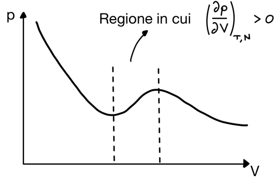
Figura 2.15: Funzione di stato con una regione in cui non vale la condizione di stabilità.
