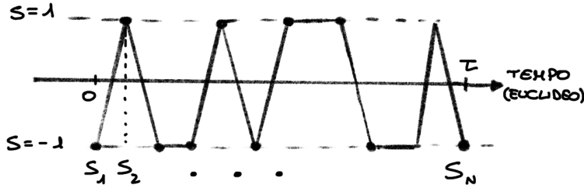
Figura 6.11: Interpretazione \hat{Z} .
