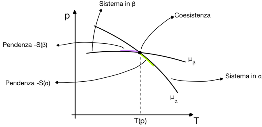
Figura 2.9: Andamento del potenziale chimico \mu in funzione della temperatura T .
