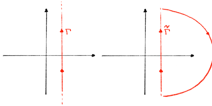
Figura 4.13: Cammini di integrazione \Gamma e \tilde{\Gamma} .
