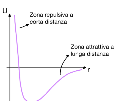
Figura 2.17: Potenziale intermolecolare.
