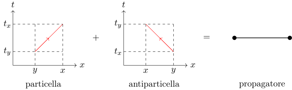
Figura 8.5: Rappresentazione propagatore di campo scalare carico.
