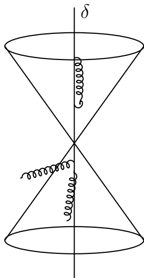
Figura 6.12: Jet con \delta finito, ma piccolo.
