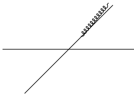
(b) Emissione di g a piccolo angolo.
