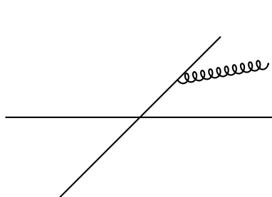
(a) Emissione di g a grande angolo.
