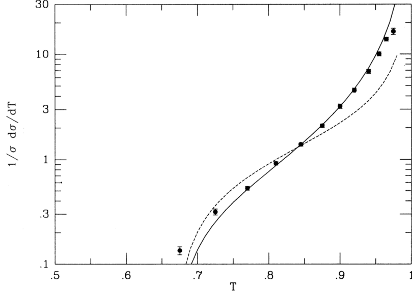
Figura 6.20: Confronto preso dall'Ellis [2]. In figura ci sono i dati sperimentali, la predizione teorica che abbiamo trovato noi (linea solida) e la predizione che si trova con una teoria di QCD scalare.
