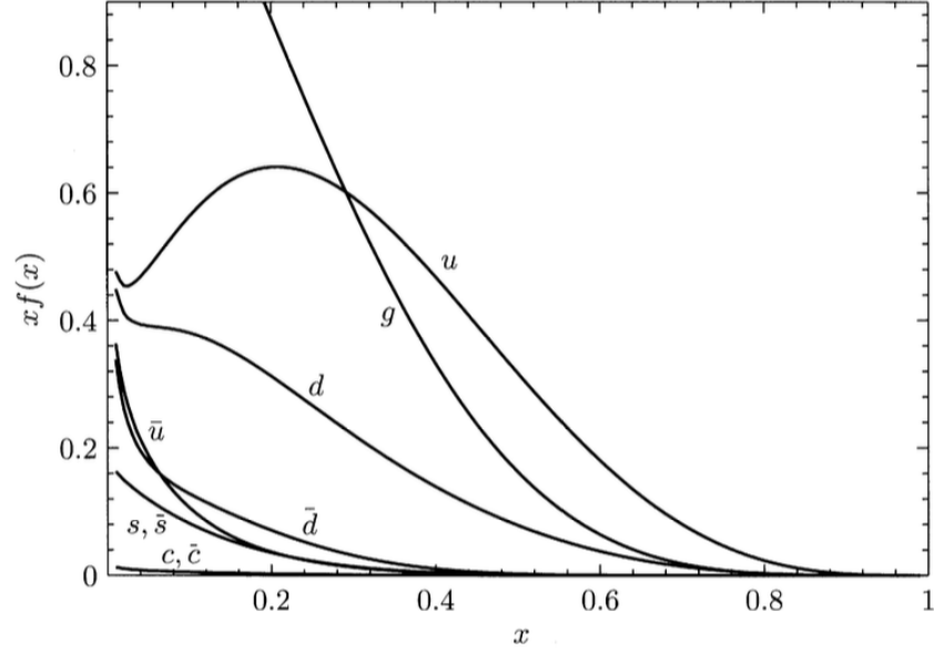
Figura 6.22: Plot preso dal Peskin [6]. Parton distribution functions x f_f(x) per quark, antiquark, e gluoni nel protone, a Q^2 = 4 \text{ GeV}^2 . Queste distribuzioni sono ottenute da un fit dei dati del deep inelastic scattering fatto dalla collaborazione CTEQ (CTEQ2L), 1993.
