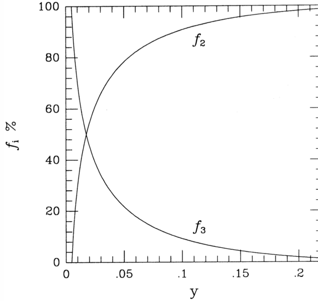
Figura 6.10: Plot di f_3 e f_2 , da Ellis [2]. Il grafico utilizza la variabile y , ma è analoga per \delta .
