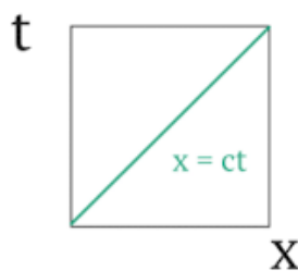
Figura 4.4: World-line fascio luminoso.
