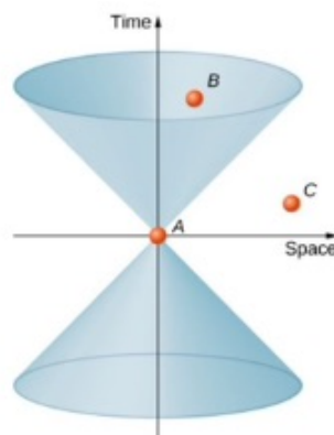
Figura 3.11: Rappresentazione cono luce di un evento A .
