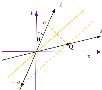
Figura 3.16: Un evento Q in due diversi sistemi di riferimento.
