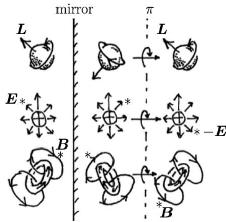
Figura 2.3: Operazione di parità su quantità fisiche. Possiamo vedere che il momento angolare \vec{L} e il campo magnetico \vec{B} si comportano come pseudovettori, ma il campo elettrico \vec{E} come un vettore.
