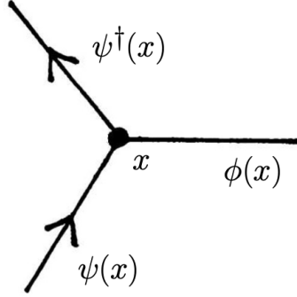
Figura 3.19: Rappresentazione vertice della teoria di Yukawa.
