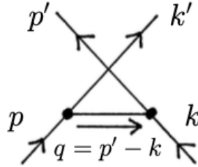
Figura 3.24: Raffigurazione canale u nello spazio degli impulsi
