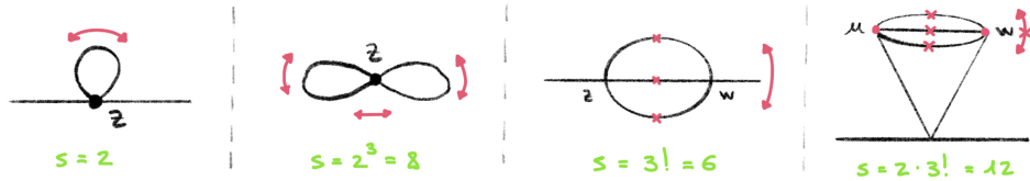
Figura 1.8: Fattori di simmetria.
