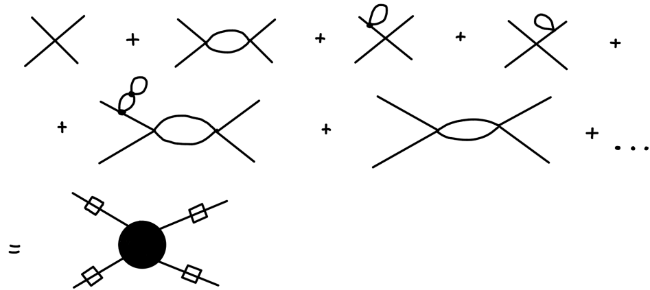
Figura 1.24: Esempio rappresentazione funzione di Green per 2 particelle iniziali e finali.
