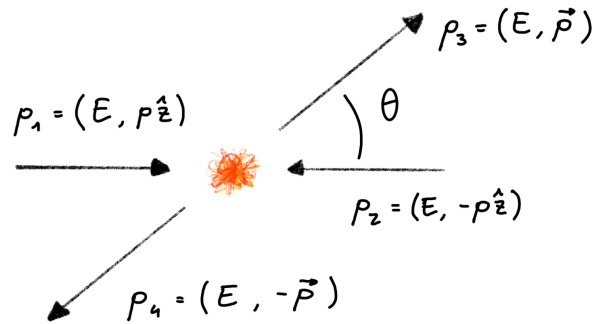
Figura 2.7: Processo d'urto 2 \rightarrow 2 .
