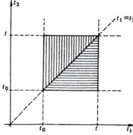
Figura 1.1: Rappresentazione geometrica dal Rossetti, Rudimenti di Meccanica Quantistica , appendice 9.
