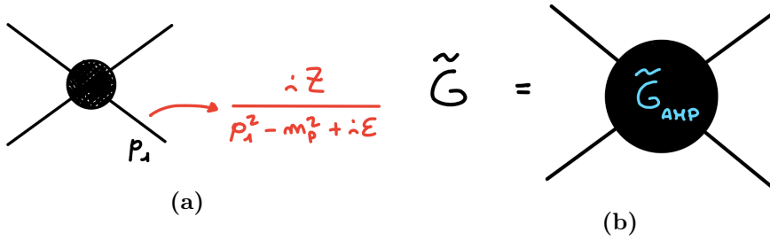
Figura 1.23: 1.23a Rappresentazione contributo linee esterne in un diagramma di Feynman. 1.23b Rappresentazione diagrammatica di \tilde{G} e \tilde{G}_{amp} . Queste immagini sono facilmente generalizzabili a diagrammi di funzioni di Green ad n + m punti (gambe esterne).
