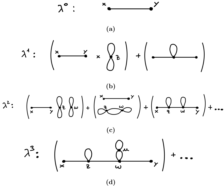
Figura 1.2: Ordini perturbativi teoria \phi^4 .
