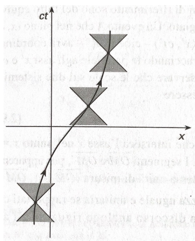
Figura 3.12: Rappresentazione con luce di diversi eventi.
