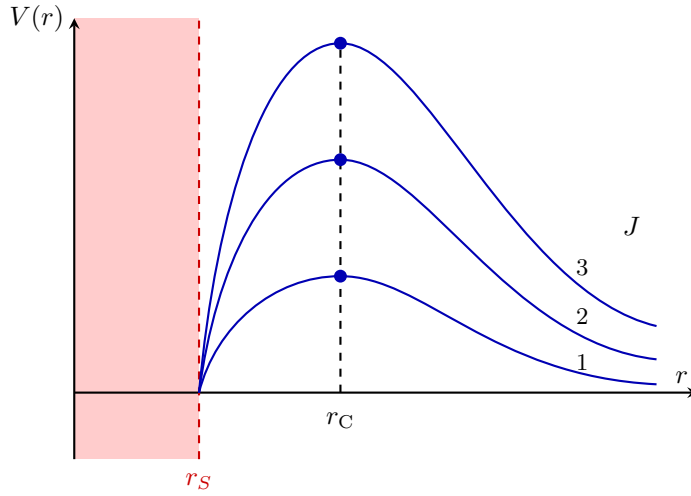
Figura 8.14: Potenziale nel caso della RG per un oggetto massless.
