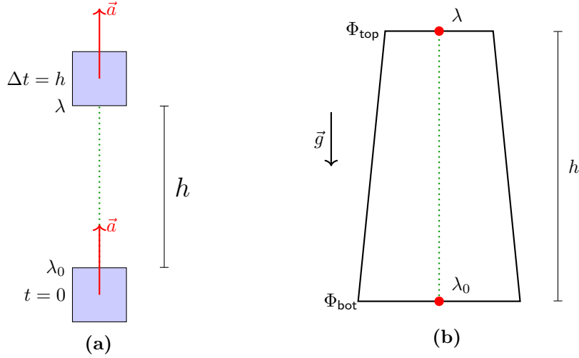
Figura 4.5: Laboratori per il redshift gravitazionale.
