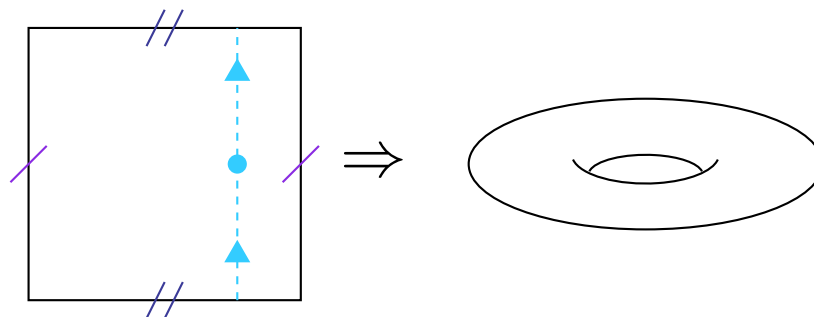
Figura 2.3: Costruzione del toro bidimensionale.
