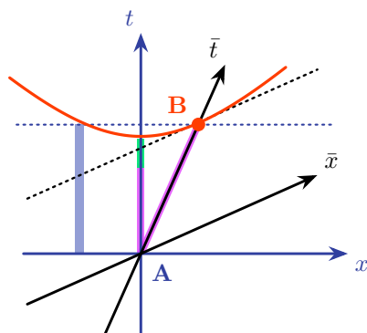
Figura 3.20: Diagramma per la dilatazione temporale.
