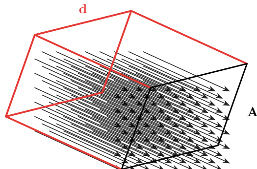
Figura 3.27: Fluido di particelle che attraversa una certa sezione.
