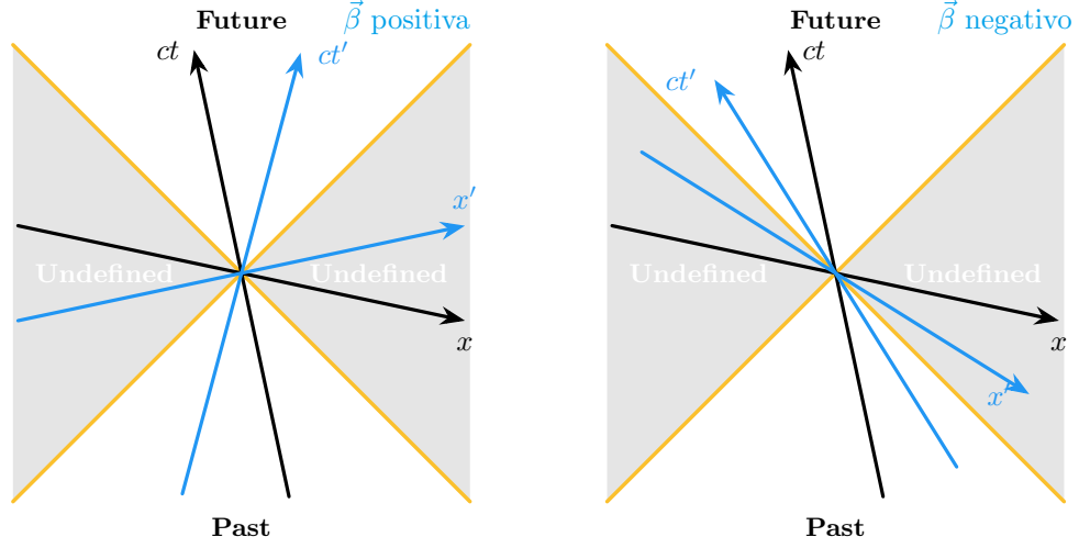
Figura 3.5: A sinistra la raffigurazione della posizione degli assi nel caso \beta > 0 , cioè in caso di moto lungo la direzione delle \hat{x} positive. A destra la raffigurazione della posizione degli assi nel caso \beta < 0 , cioè in caso di moto lungo la direzione delle \hat{x} negative.
