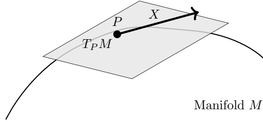
Figura 2.2: Piano tangente al punto P della varietà M .
