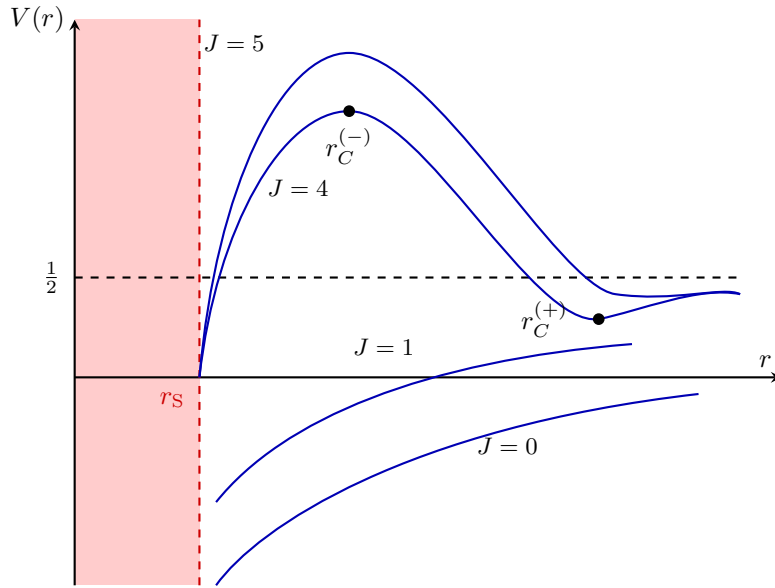
Figura 8.16: Potenziale nel caso della RG per un oggetto massivo.
