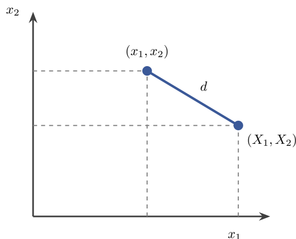
Figura 2.1: Distanza euclidea.
