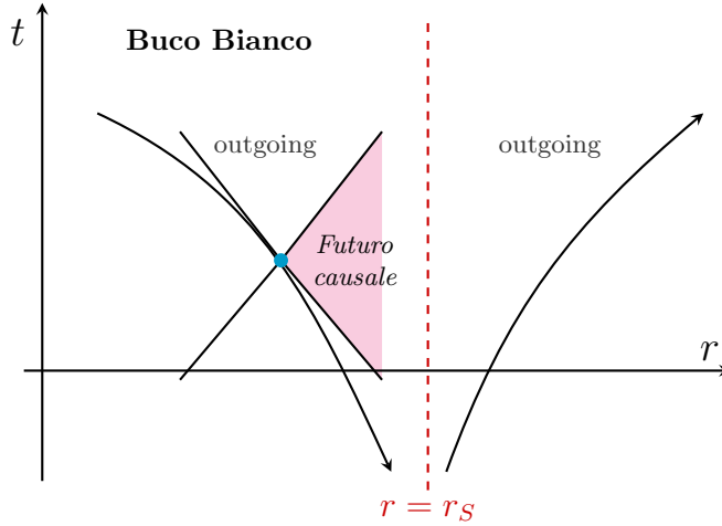
(b) Rappresentazione worldline outgoing, descritte dalle equazioni (8.1.57).
