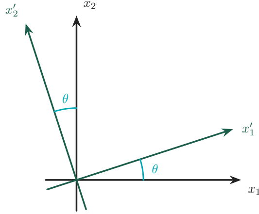
Figura 3.3: Diagramma spaziale.
