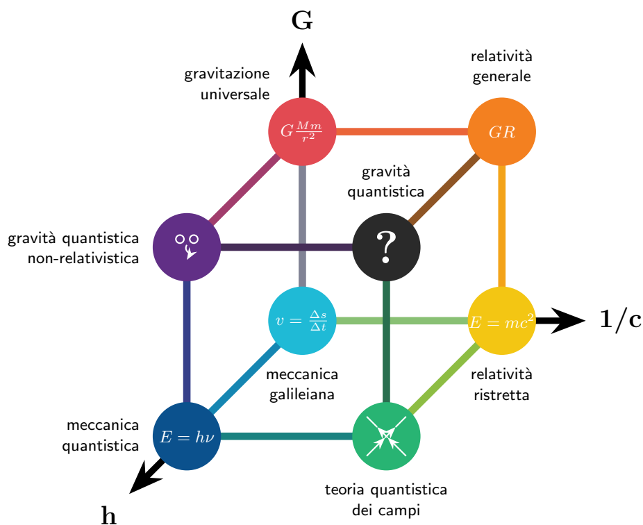
Figura 1.2: Cubo delle teorie di Zelmanov.
