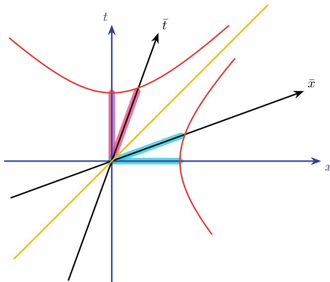
Figura 3.19: Sistemi di riferimento O e O' insieme alle iperboli invarianti.
