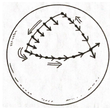
Figura 2.8: Trasporto parallelo su una superficie curva bidimensionale.
