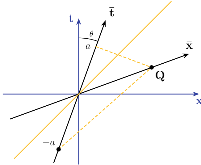
Figura 3.15: Un evento Q in due diversi sistemi di riferimento.
