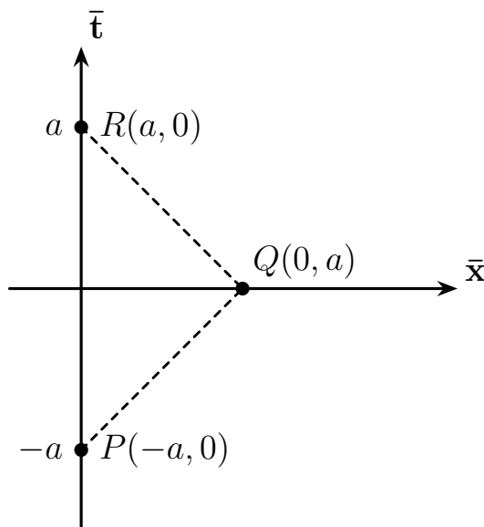
Figura 3.16: Costruzione asse \bar{x} .
