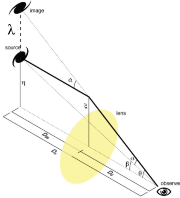
Figura 7.4: Lente gravitazionale in approssimazione di lente sottile.
