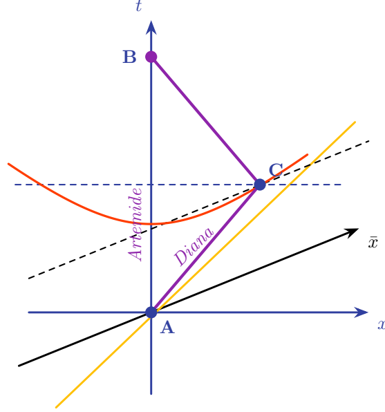
Figura 3.22: Paradosso dei gemelli.
