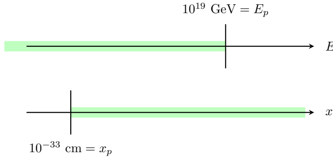
Figura 1.1: Rappresentazione scala di Planck.
