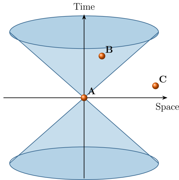
Figura 3.11: Rappresentazione cono luce di un evento A .
