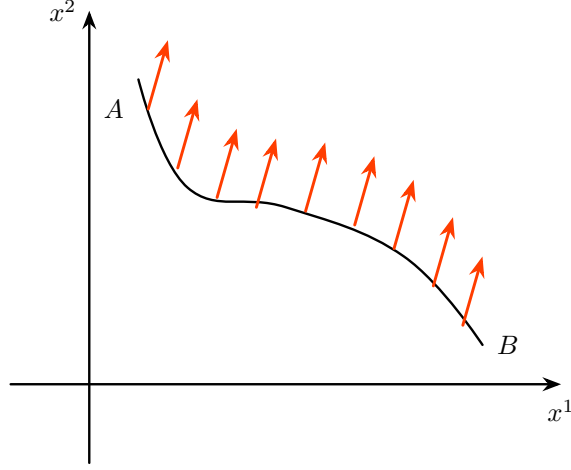
Figura 5.1: Trasporto parallelo in uno spazio piatto.
