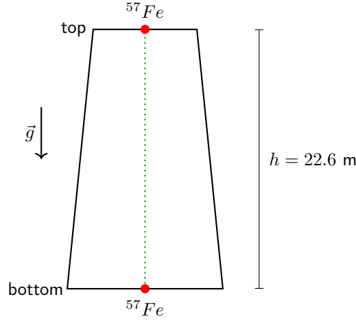
Figura 4.8: Set up sperimentale esperimento di Pound e Rebka.
