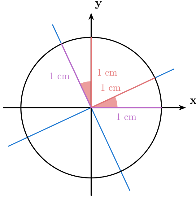
Figura 3.17: Calibrazione nel piano euclideo.
