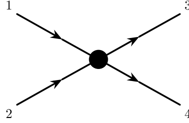
Figura 3.26: Processo d'urto.
