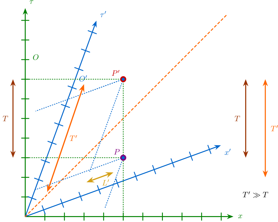
Figura 3.21: Diagramma per la dilatazione temporale.
