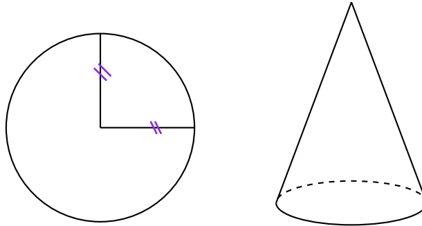
Figura 2.5: Raffigurazione cono.
