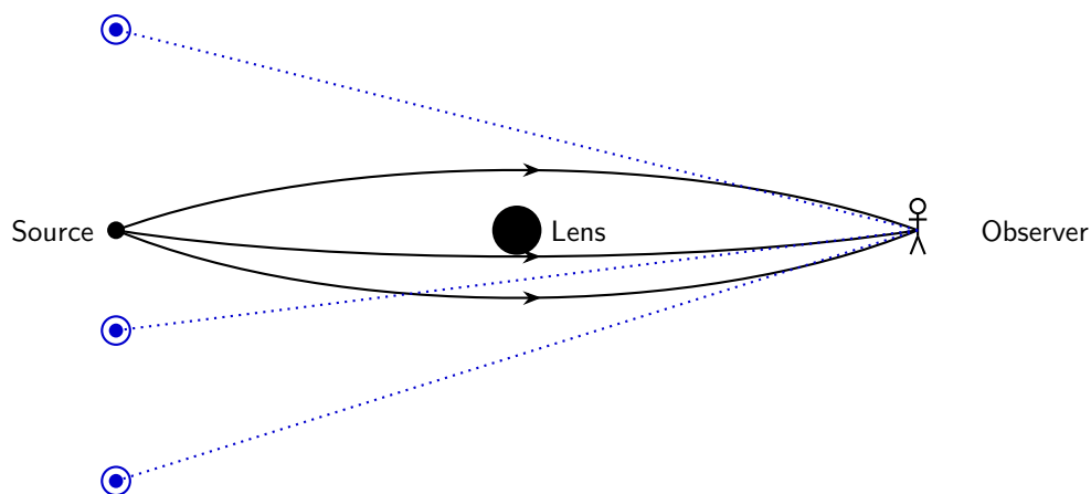
(a) Rappresentazione lente gravitazionale.
