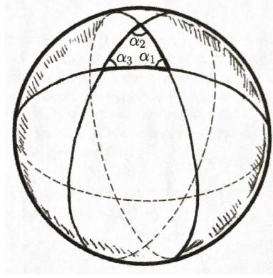
Figura 2.6: Triangolo costruito su una superficie curva.
