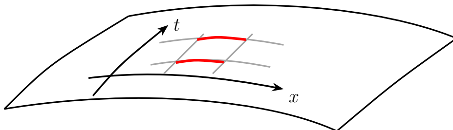
Figura 4.7: Laboratori per il redshift gravitazionale in uno spaziotempo curvo. I tratti arancioni, in uno spazio curvo, potrebbero non essere uguali.
