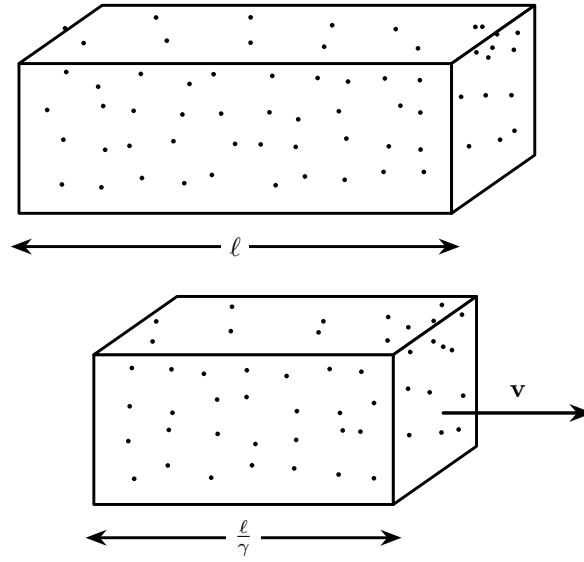
Figura B.1: Contrazione dei volumi.
