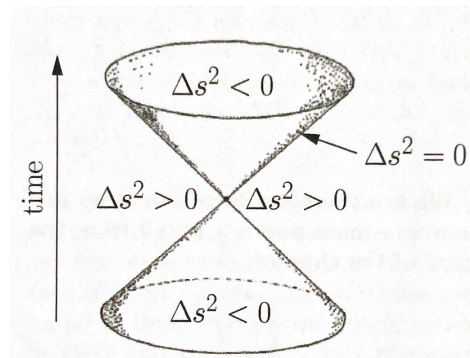
(b) Intervalli sul cono luce.
