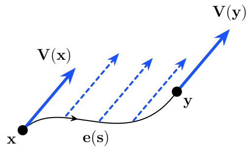
Figura 2.7: Trasporto parallelo.
