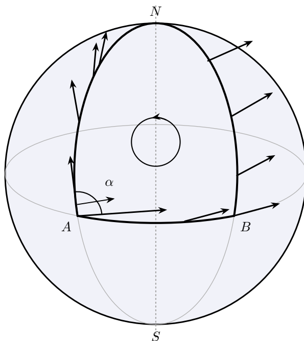
Figura 5.2: Trasporto parallelo in uno spazio curvo.
