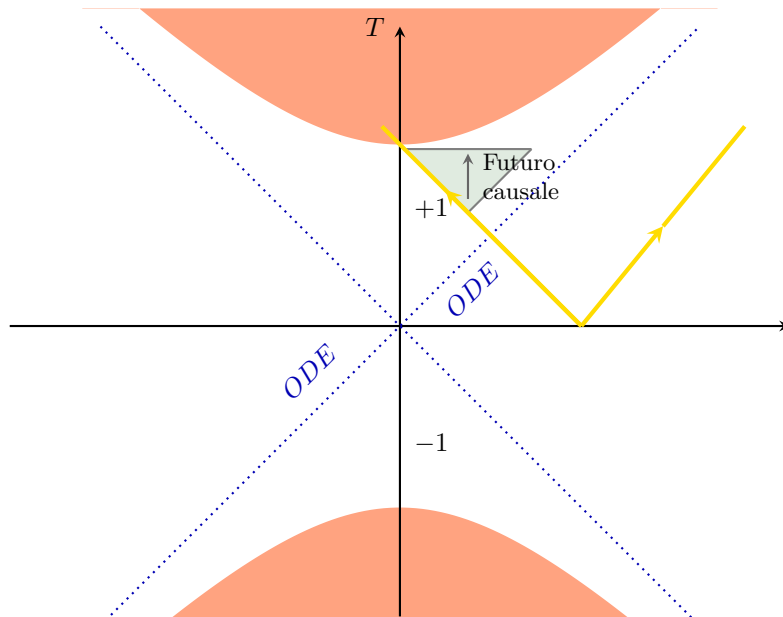
Figura 8.20: Rappresentazione di un fotone, visto da un osservatore nelle coordinate (T, R) , che entra nel buco nero.
