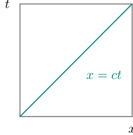
Figura 4.4: World-line fascio luminoso.
