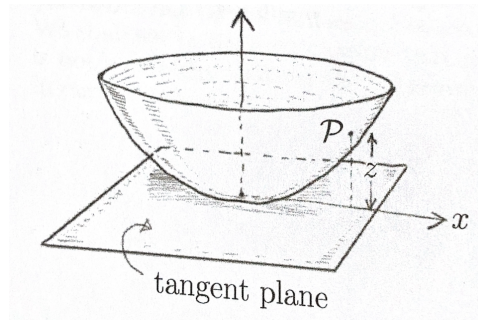
Figura 4.3: Rappresentazione piano tangente ad una varietà curva.
