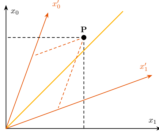
Figura 3.4: Diagramma spaziotemporale.
