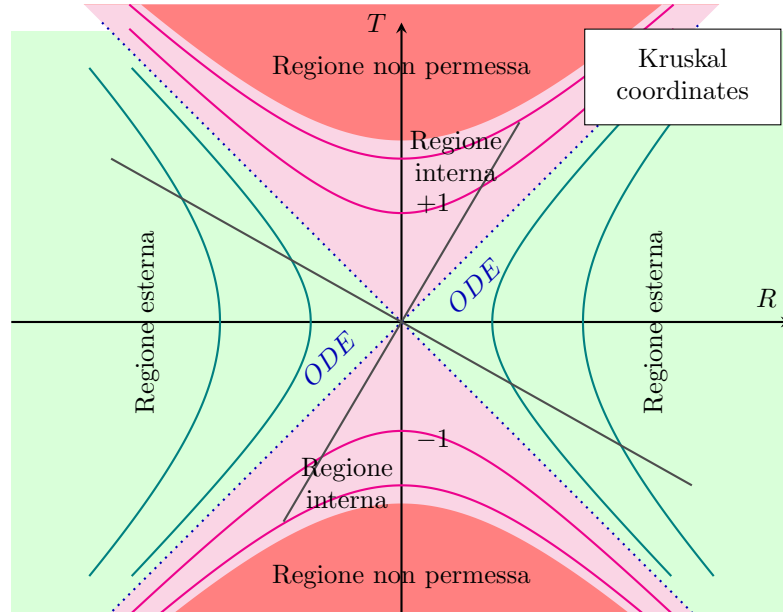
Figura 8.19: Spaziotempo nelle coordinate di Kruskal.
