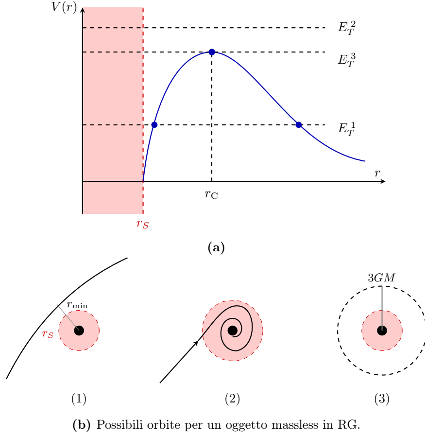
Figura 8.15: Studio delle possibili orbite per una particella massless in RG.
