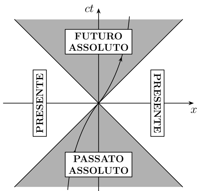
Figura 3.13: Rappresentazione passato e futuro di un evento.
