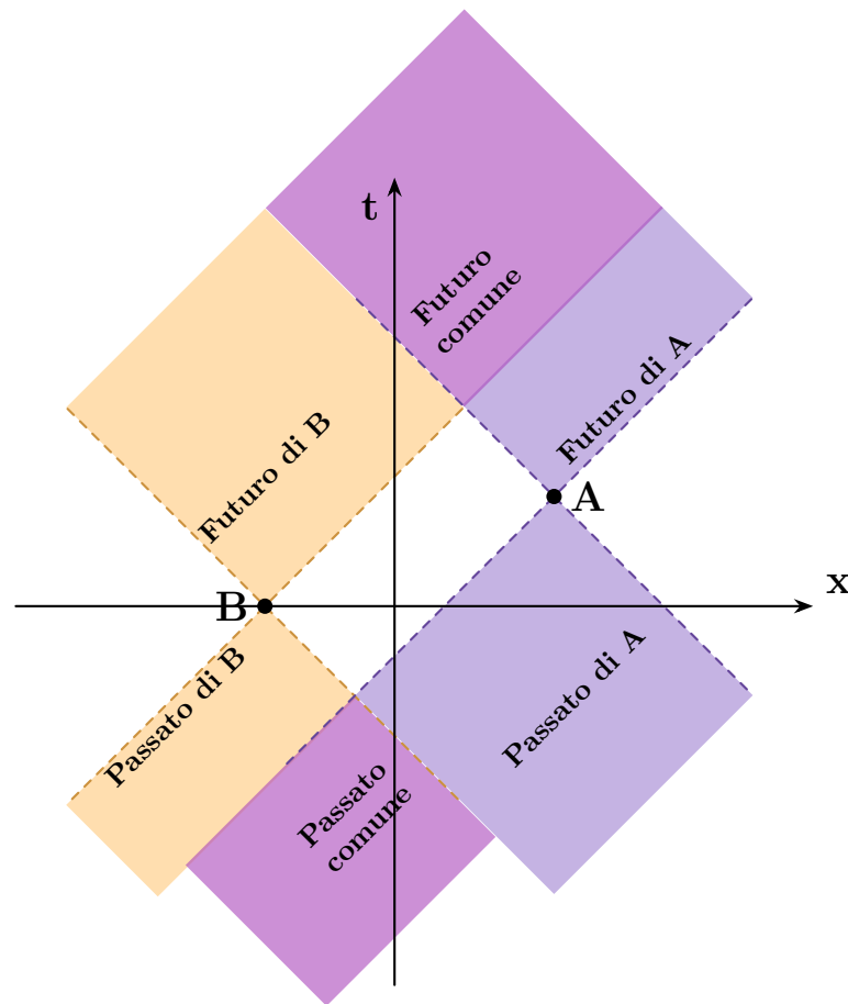
Figura 3.10: Rappresentazione passato e futuro di un evento.
