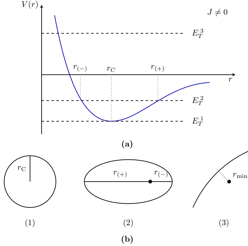
Figura 8.13: Rappresentazione moti orbitali con J \neq 0 .
