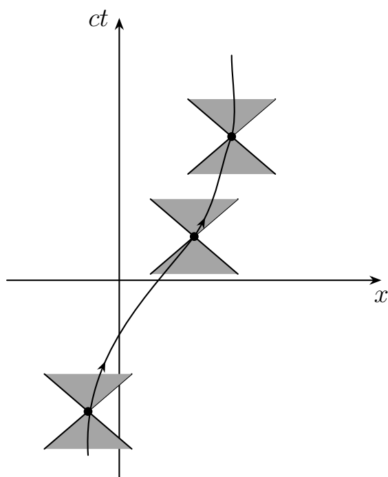
Figura 3.12: Rappresentazione cono luce di diversi eventi.
