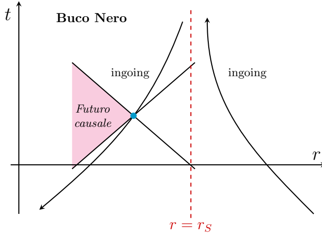
(a) Rappresentazione worldline ingoing, descritte dalle equazioni (8.1.56).
