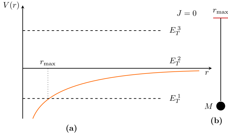
Figura 8.12: Rappresentazione moti orbitali con J = 0 .
