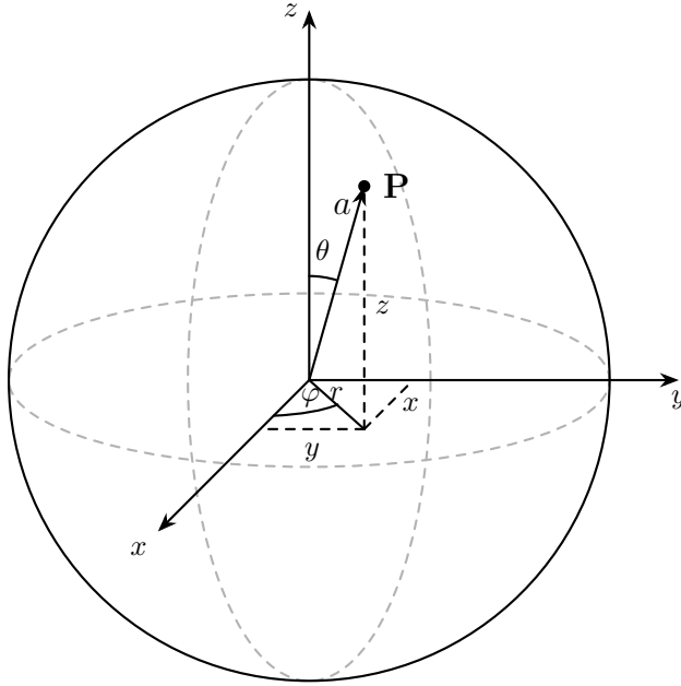
Figura A.1: Superficie sferica \mathbb{S}^2 nello spazio di immersione \mathbb{R}^3 . Indichiamo nell'immagine (x, y, z) = (x_1, x_2, x_3) e il raggio r = a .
