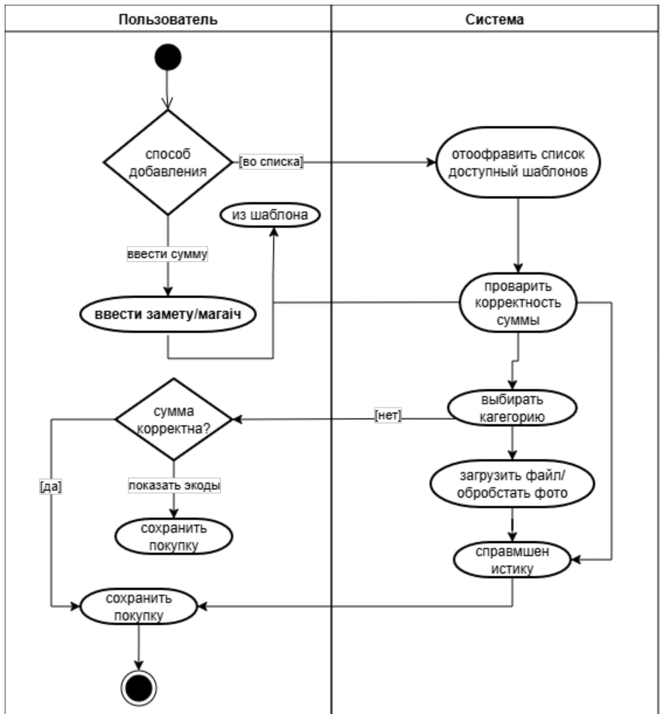
Рисунок 3.1 — Диаграмма активности варианта использования «Добавление покупки»
